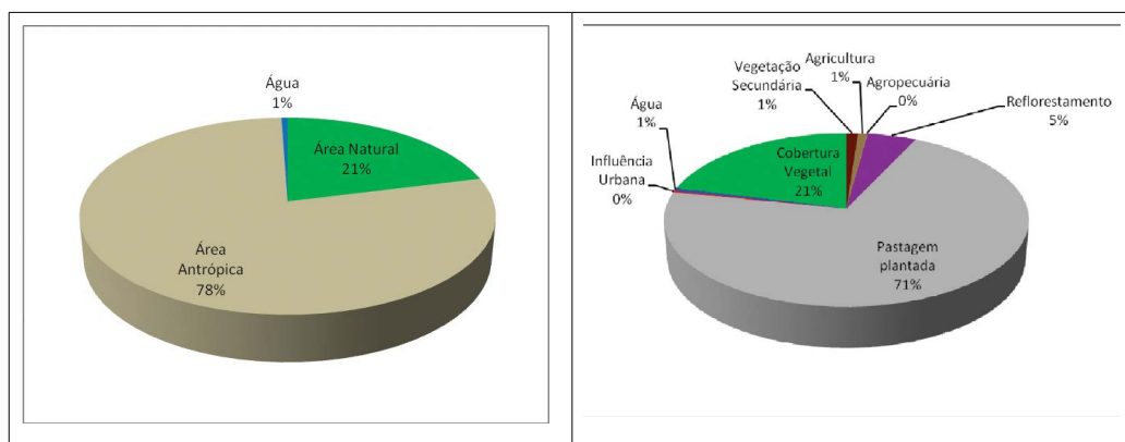
Figura 3a. Predomínio da área antrópica em relação a área natural; Figura 3b. Quantificação do uso e cobertura da terra
