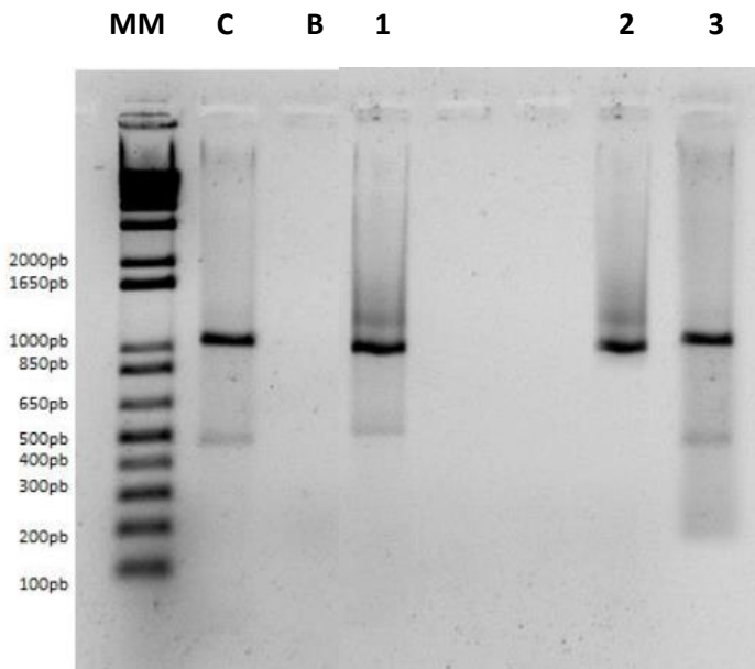
Figura 3. Amostras de sorgo selvagem (1), teosinto (2) e capim marmelada (3) apresentando amplicon de 1072 pb, resultante da amplificação com o par de primers (MDMV2/MDMV3) que amplifica a sequência do gene da proteína capsidial de SCMV. Gel de agarose 1,5%. MM= marcador molecular, C= controle e B=branco.
