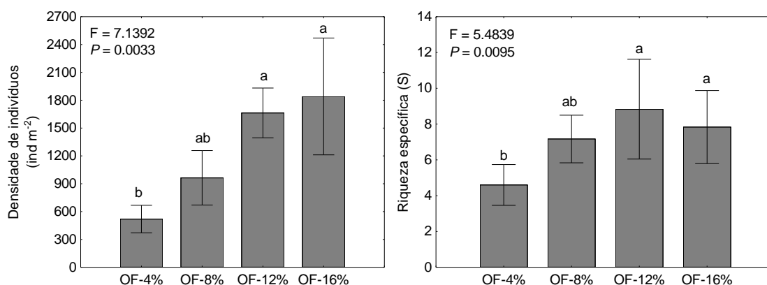
Figura 4.3. Médias e desvios padrões da densidade de indivíduos e da riqueza específica de colêmbolo em quatro níveis de oferta de forragem (4%, 8%, 12% e 16%). Diferentes letras significam diferença estatística ( p < 0,05 , Tukey HSD).
