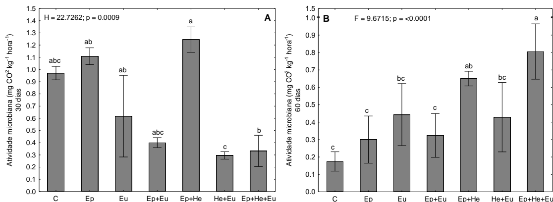
Figura 5.2. Médias e desvios padrões da atividade microbiana do solo medida a partir da evolução de CO 2 aos 30 e 60 dias após introdução dos colêmbolos. Diferentes letras denotam diferença estatística ( P < 0,05 , Tukey HSD). Nenhuma letra denota ausência de diferença significativa. Ver legenda na Tabela 5.1.
