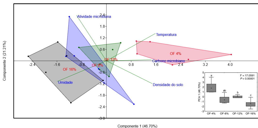
Figura 4.2. Análise de componentes principais e análise de variância do primeiro eixo de ordenação dos fatores bióticos e abióticos do solo em quatro níveis de oferta de forragem (4%, 8%, 12% e 16%).
