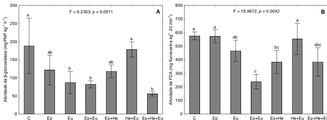
Figura 5.3. Média e desvios padrões da atividade enzimática da \beta -glucosidase e FDA 60 dias após introdução dos colêmbolos. Diferentes letras denotam diferença estatística ( P < 0,05 , UNEQUAL N HSD). Nenhuma letra denota ausência de diferença significativa. Ver legenda na Tabela 5.1.
