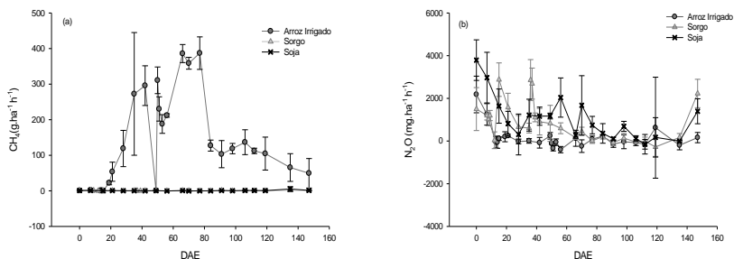
Figura 1. Fluxos de CH 4 (a) e de N 2 O (b) em Planosolo cultivado com arroz irrigado, soja e sorgo forrageiro. Barras verticais representam o desvio padrão da média.
