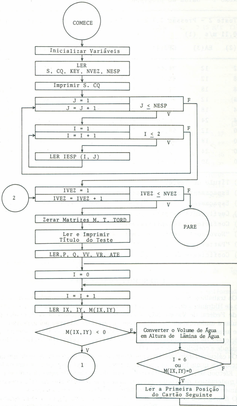
FIGURA 5 - Fluxograma que demonstra a lógica do programa.
