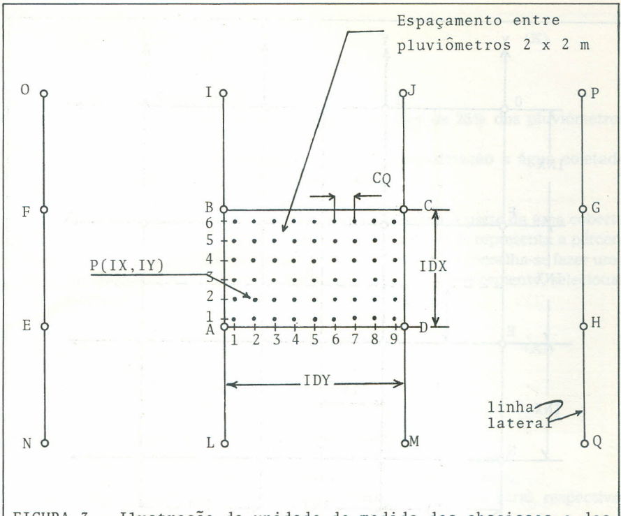
FIGURA 3 - Ilustração da unidade de medida das abscissas e das ordenadas. As letras A a Q representam os aspersores, P(IX,IY) representa o pluviômetro de coordenadas IX e IY, IDY é o espaçamento entre as linhas laterais, IDX é o espaçamento entre os aspersores ao longo da linha lateral e CQ é o comprimento da quadrícula.
