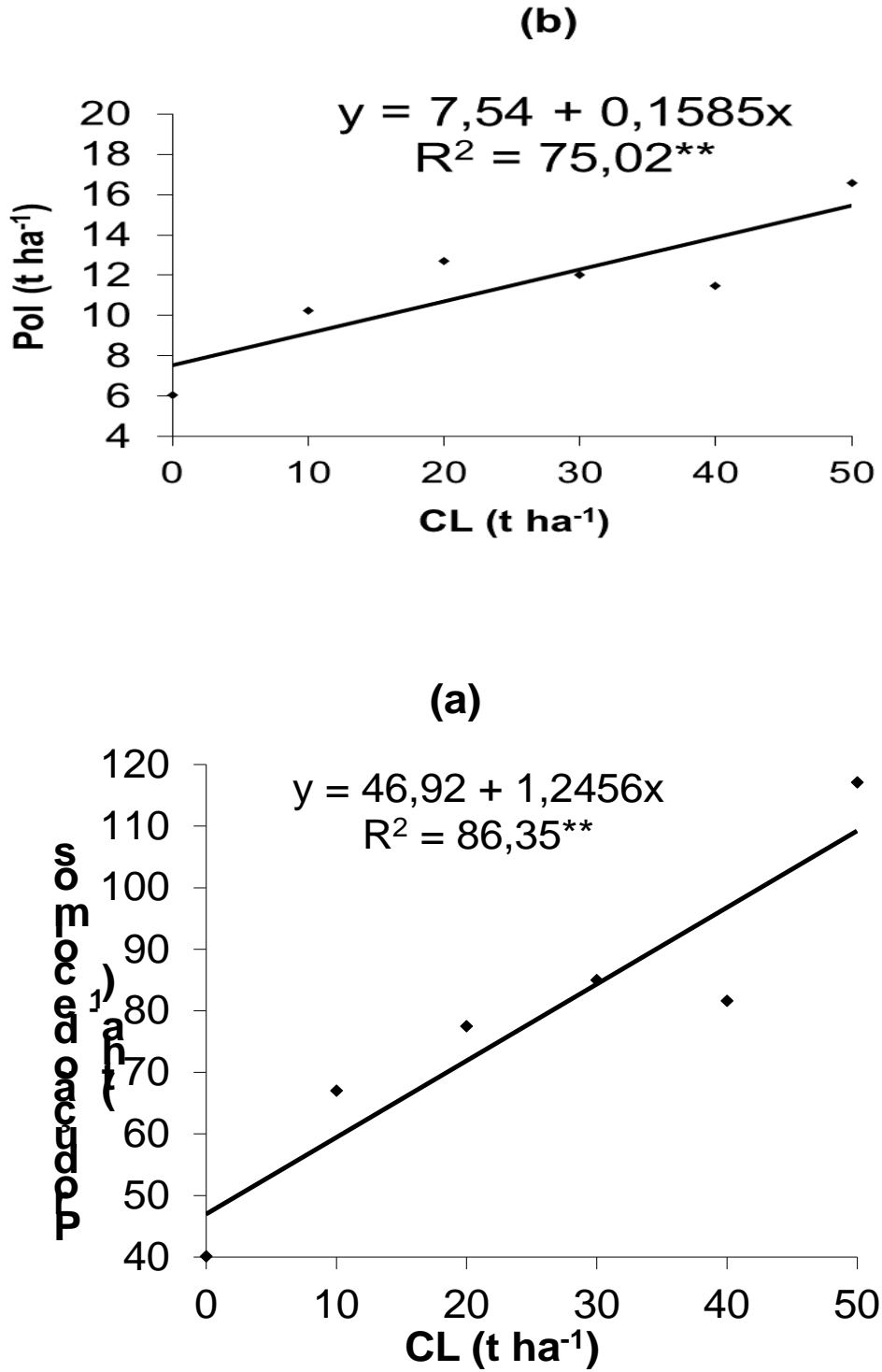
Figura 3. Influência da aplicação de composto de lixo na produtividade de colmos (a) e de açúcar (b) por hectare na cana-planta já adubada com NPK.
