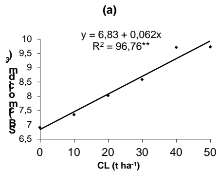
Figura 2. Influência da aplicação de composto de lixo na soma de bases (a) e na saturação por bases (b) aos 120 dias após plantio em solo já adubado com NPK.
