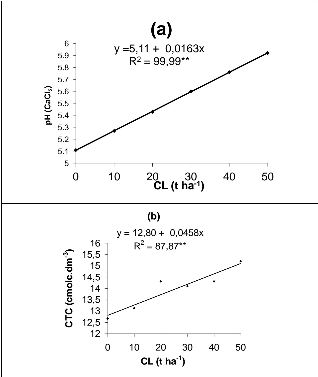
Figura 1. Influência da aplicação de composto de lixo no \text{pH}_{\text{CaCl}_2} (a) e na capacidade de troca catiônica (CTC) do solo (b) aos 120 dias após plantio em solo já adubado com NPK.
