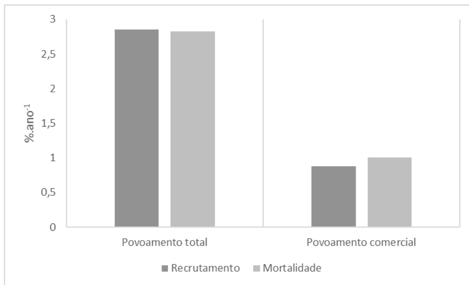
Figura 13. Balanço dinâmico do povoamento geral considerando um tempo médio de 17 anos, para todas as espécies e para as espécies comerciais/potenciais em 8,2 hectares amostrados de uma Floresta Ombrófila Densa sob regime de Manejo Florestal da empresa Mil Madeiras, Itacoatiara-AM.
