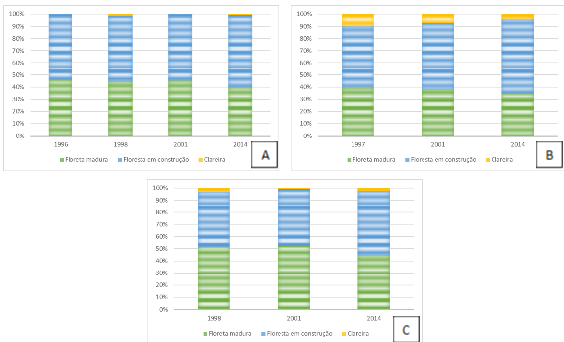
Figura 18. Percentual das classes de floresta, antes da exploração (B-1996; C-1997; D-1998) e após a exploração (B-1998, 2001 e 2014; C-2001 e 2014; D-2001 e 2014), nos 8,2 hectares amostrados de uma Floresta Ombrófila Densa pertencente a área de Manejo Florestal da empresa Mil Madeiras, Itacoatiara-AM. Figura A = compartimento B, Figura B = compartimento C, Figura C = compartimento D.
