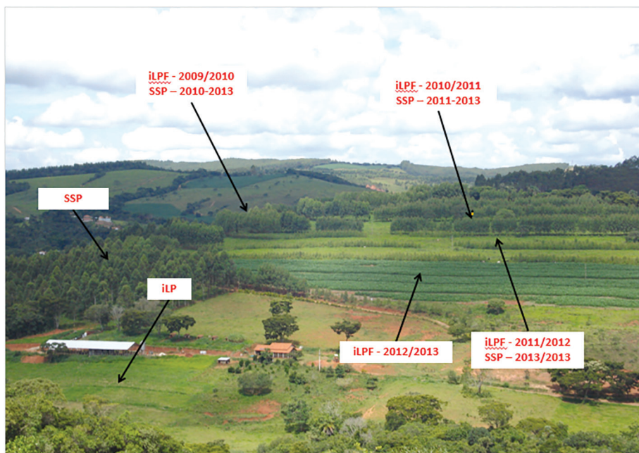
Figura 6. URT ILPF da Embrapa Gado de Leite com o consórcio eucalipto/milho/capim e sequência de implantação em glebas anuais – Fase Agrossilvicultural.
