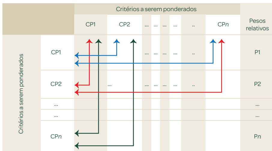
Figura 2. Ilustração da aplicação do método AHP para hierarquização de critérios na matriz de comparação pareada.
