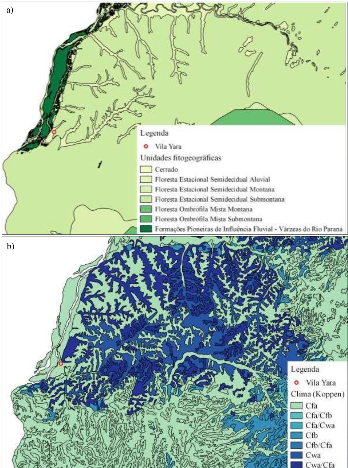
Figura 03: Caracterização física da área de estudo. a) unidades fitogeográfica; b) clima.
