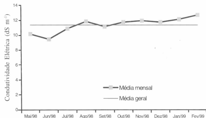
Figura 1. Comportamento da salinidade da água do rejeito da dessalinização
