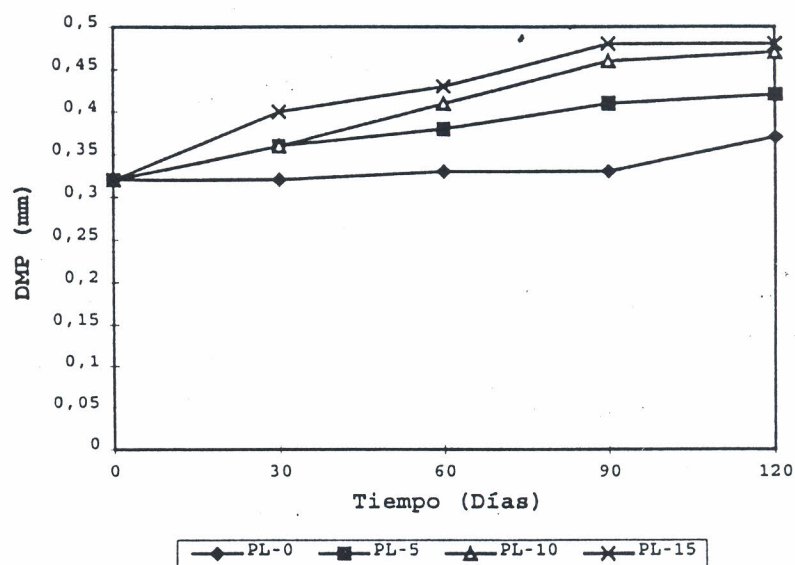
Figura 2. Variación del DMP en el suelo PL, respecto las dosis de polímero aplicadas y el tiempo.
