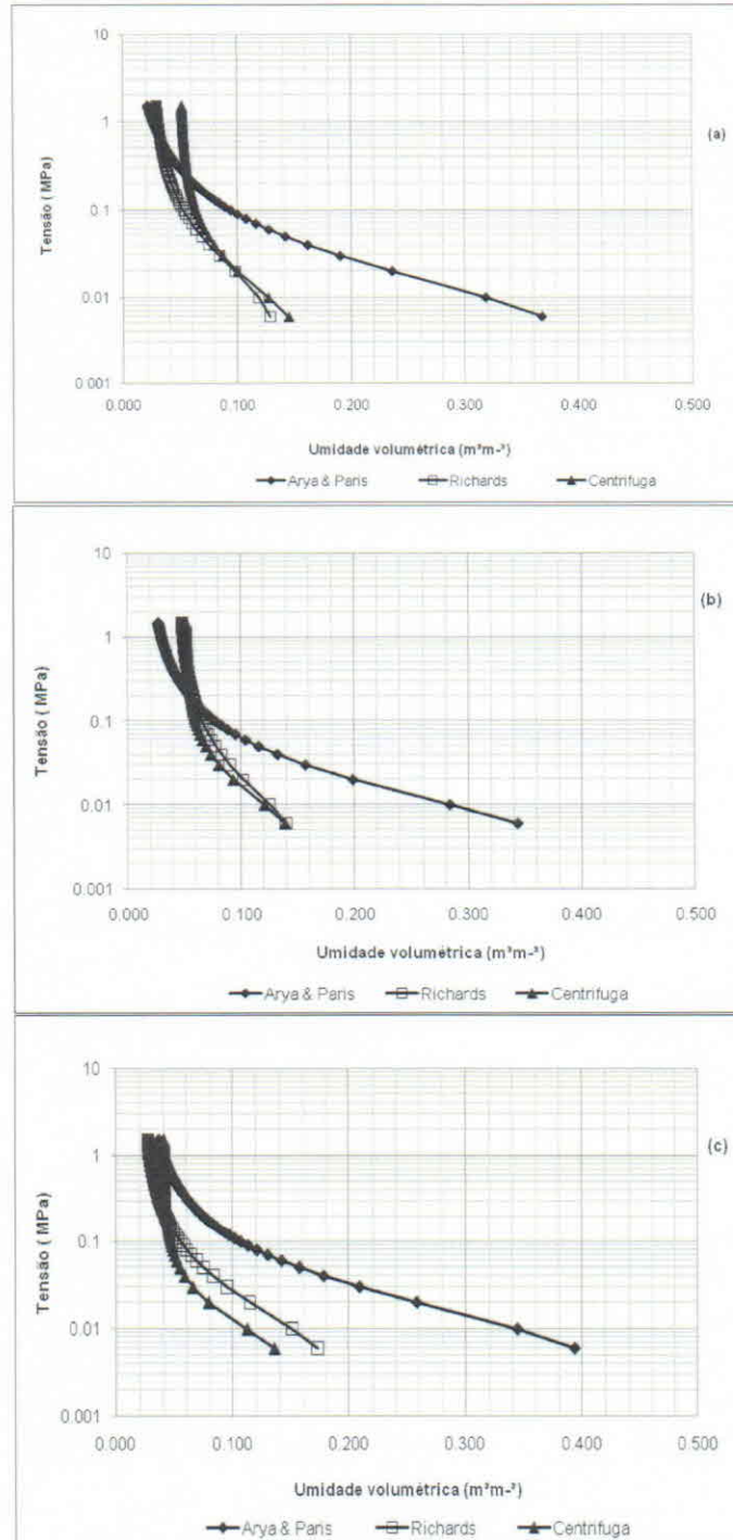
Figura 1. Curvas de retenção obtidas pelos métodos Arya & Paris (AP), câmara de Richards (R) e centrífuga (C), nas camadas de 0,0-0,20 m (a); 0,20-0,40 m (b) e 0,40-0,60 m (c) de profundidade.
