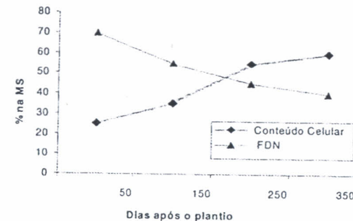
FIGURA 2 - Variação na composição da cana-de-açúcar em função da idade da planta (PATE, 1977).
