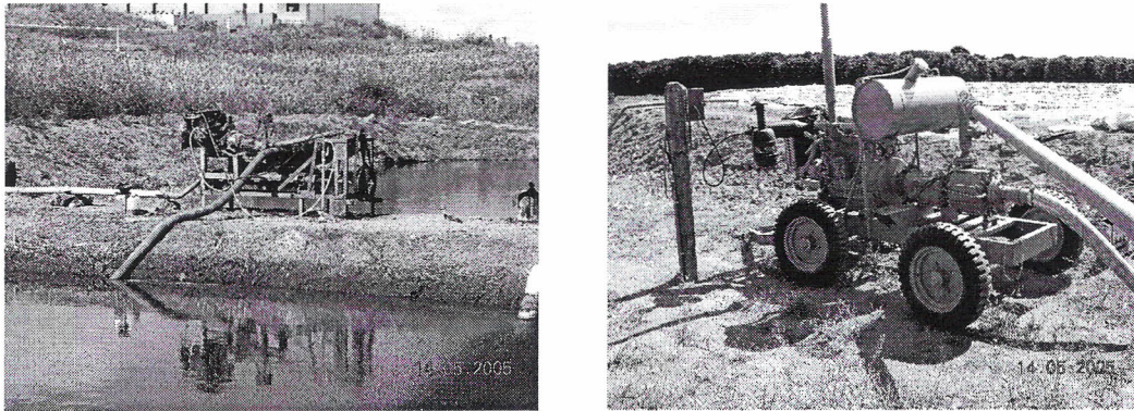
Fig. 6. Transferência do biofertilizante com motor gasolina/biogás (A) e aplicação no campo via autopropelido com motor diesel/biogás (B)
