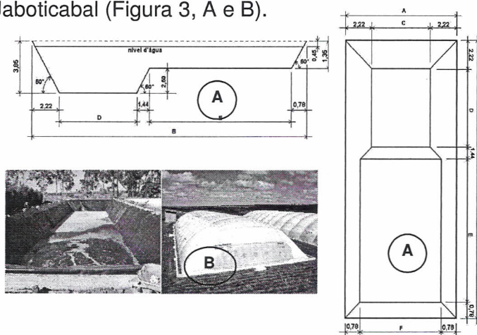
Fig. 3. Modelo de biodigestor adotado pela empresa AgCert, em planta baixa (A) e construído (B).
