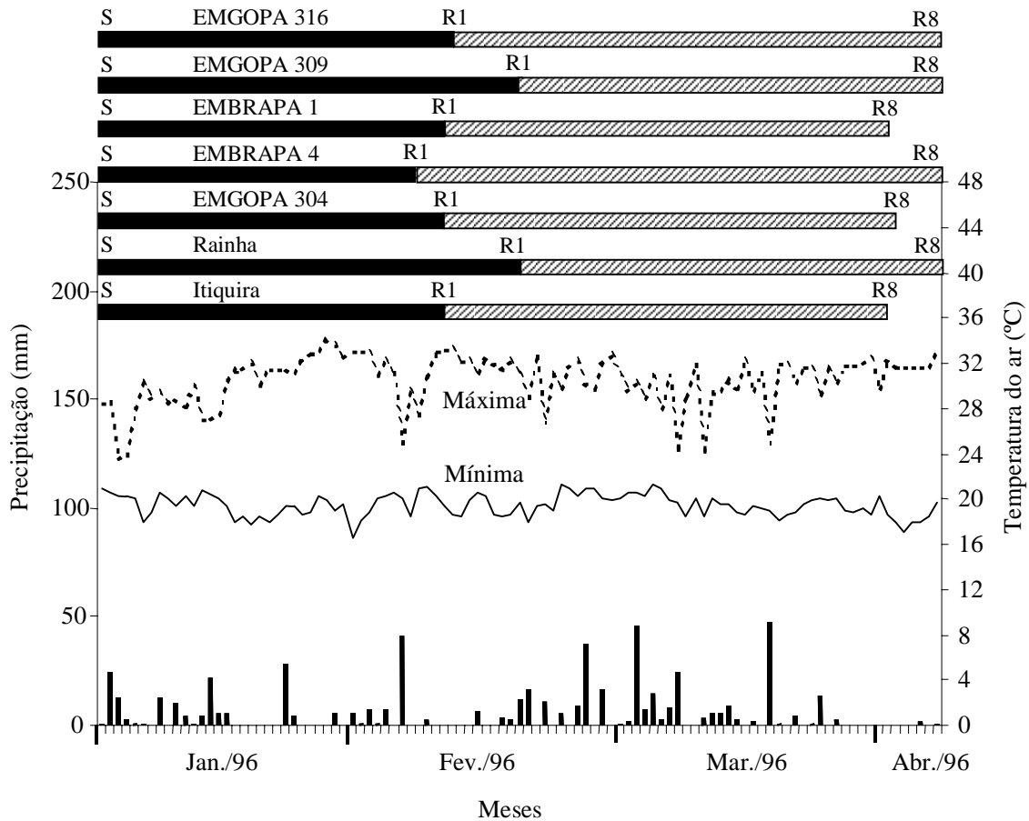
FIG. 3. Época de semeadura (30/12/95): ciclos culturais e estádios fenológicos das plantas de soja (S = semeadura; R1, R8 = estádios reprodutivos); dados diários de precipitação pluvial e de temperaturas máxima e mínima. Goiânia, GO.
