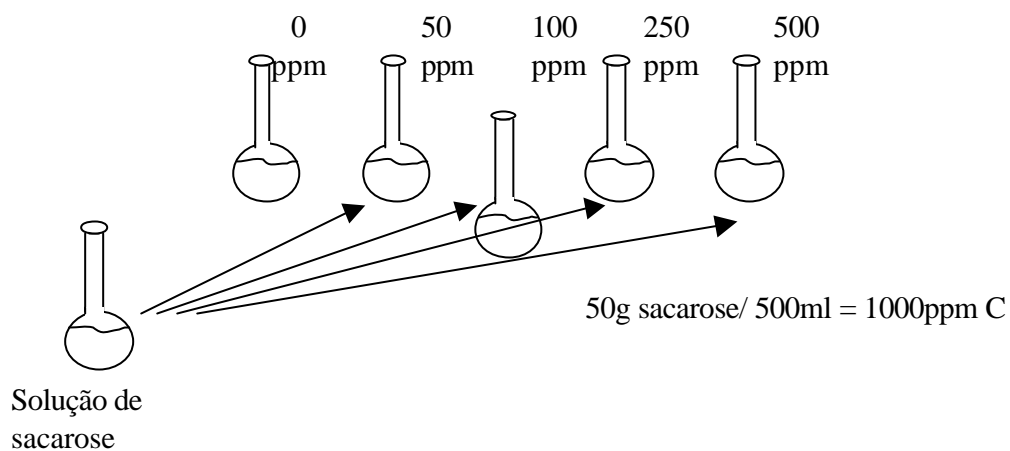
Figura 9 – Esquema para obter soluções com concentração de carbono conhecida.
