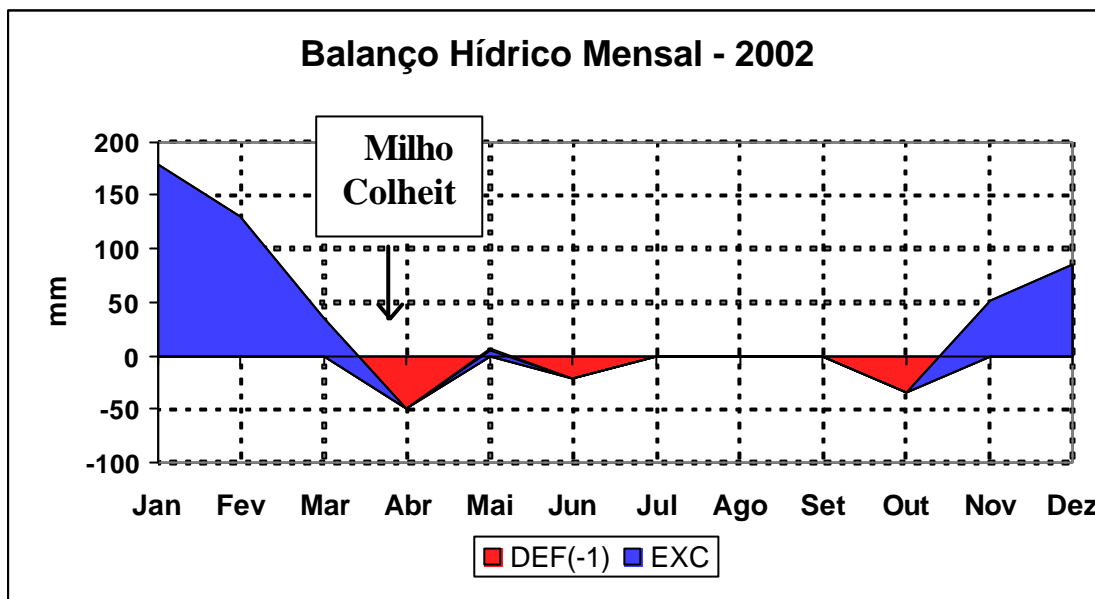
Figura 5- Balanço hídrico verificado na Fazenda Experimental Lageado no ano de 2002.
