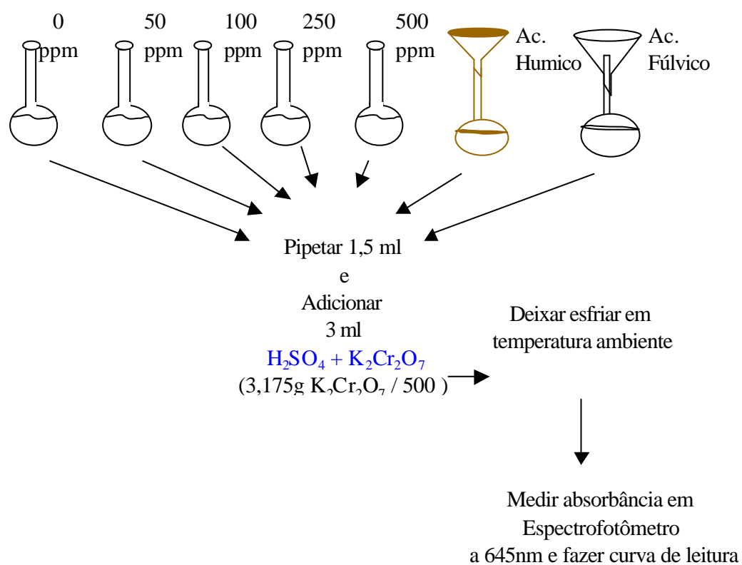
Figura 10- Esquema para determinação dos ácidos húmicos e fúlvicos da matéria orgânica do solo.
