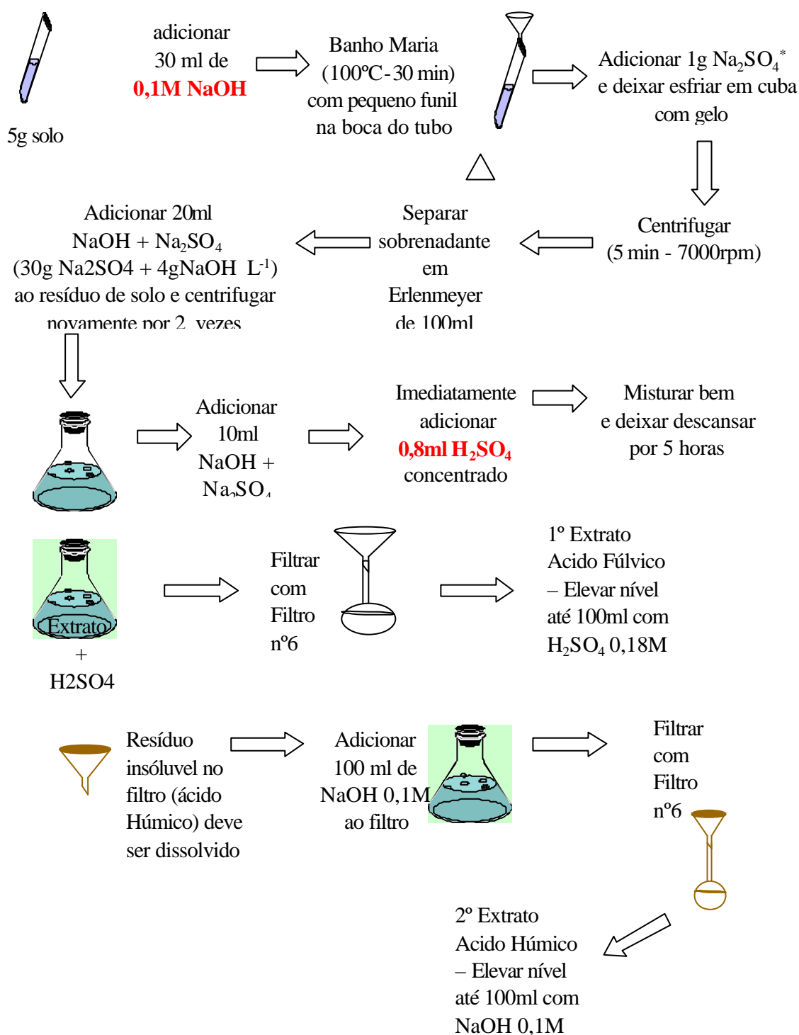
Figura 8 – Esquema de extração dos ácidos húmicos e fúlvicos da matéria orgânica do solo.
