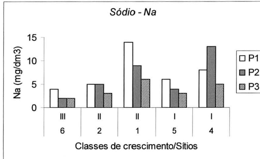
FIGURA 4.4 - TEOR DE SÓDIO ( \text{mg}/\text{dm}^3 ) NAS PARCELAS DE SCLEROLOBIUM PANICULATUM , AOS 24 MESES DE IDADE, NAS PROFUNDIDADES P1 (0-20 cm), P2 (20-40 cm), P3 (40-80 cm)
