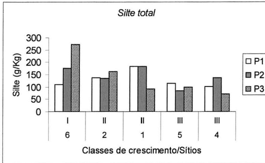
FIGURA 4.19 - TEOR DE SILTE (g/Kg) NAS PARCELAS DE SCLEROLOBIUM PANICULATUM , AOS 24 MESES DE IDADE, NAS PROFUNDIDADES P1 (0-20 cm), P2 (20-40 cm), P3 (40-80 cm)
