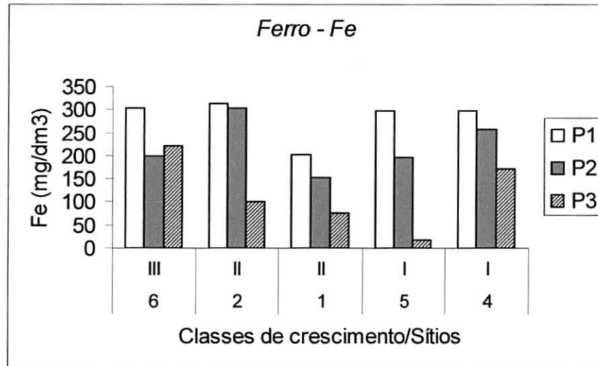
FIGURA 4.6 - TEOR DE FERRO ( \text{mg}/\text{dm}^3 ) NAS PARCELAS DE SCLEROLOBIUM PANICULATUM , AOS 24 MESES DE IDADE, NAS PROFUNDIDADES P1 (0-20 cm), P2 (20-40 cm), P3 (40-80 cm)
