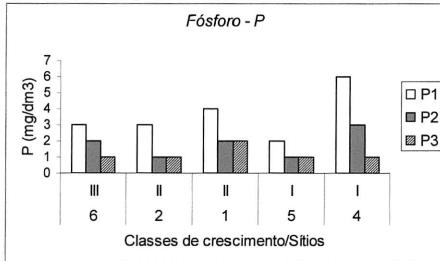
FIGURA 4.8 - TEOR DE FÓSFORO ( \text{mg}/\text{dm}^3 ) NAS PARCELAS DE SCLEROLOBIUM PANICULATUM , AOS 24 MESES DE IDADE, NAS PROFUNDIDADES P1 (0-20 cm), P2 (20-40 cm), P3 (40-80 cm)
