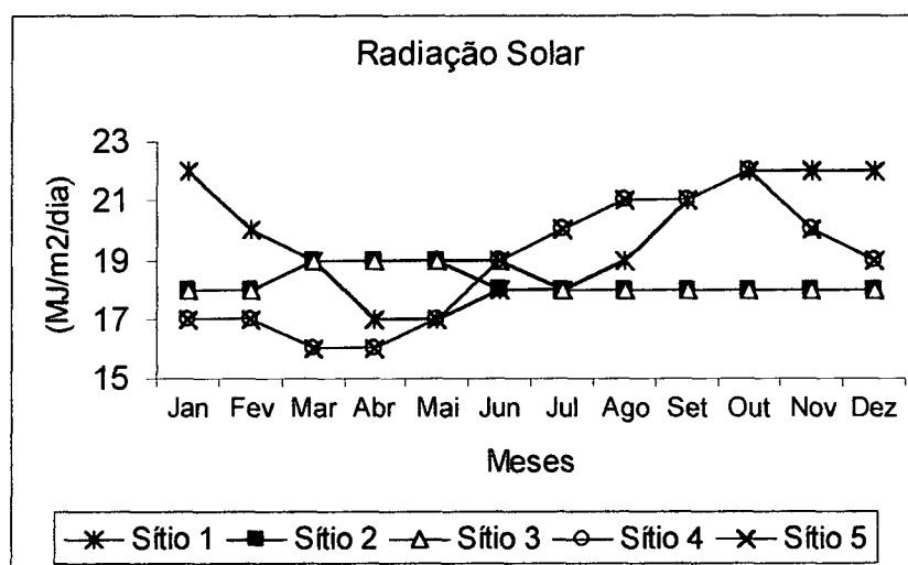
FIGURA 4.33 - RADIAÇÃO SOLAR (MJ/m 2 /dia) EM CINCO SÍTIOS NA AMAZÔNIA, ESTIMADA A PARTIR DAS COORDENADAS GEOGRÁFICAS
