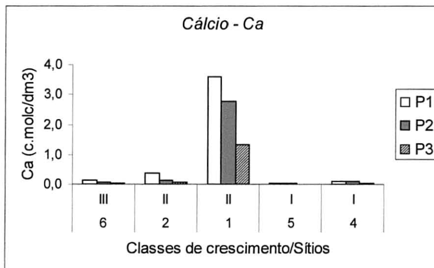
FIGURA 4.11 - TEOR DE CÁLCIO (c.molc/dm 3 ) NAS PARCELAS DE SCLEROLOBIUM PANICULATUM , AOS 24 MESES DE IDADE, NAS PROFUNDIDADES P1 (0-20 cm), P2 (20-40 cm), P3 (40-80 cm)
