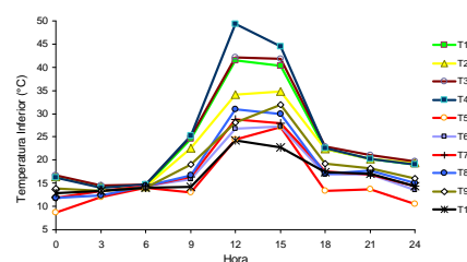
Figura 3. Gráfico da temperatura inferior das cortinas.
