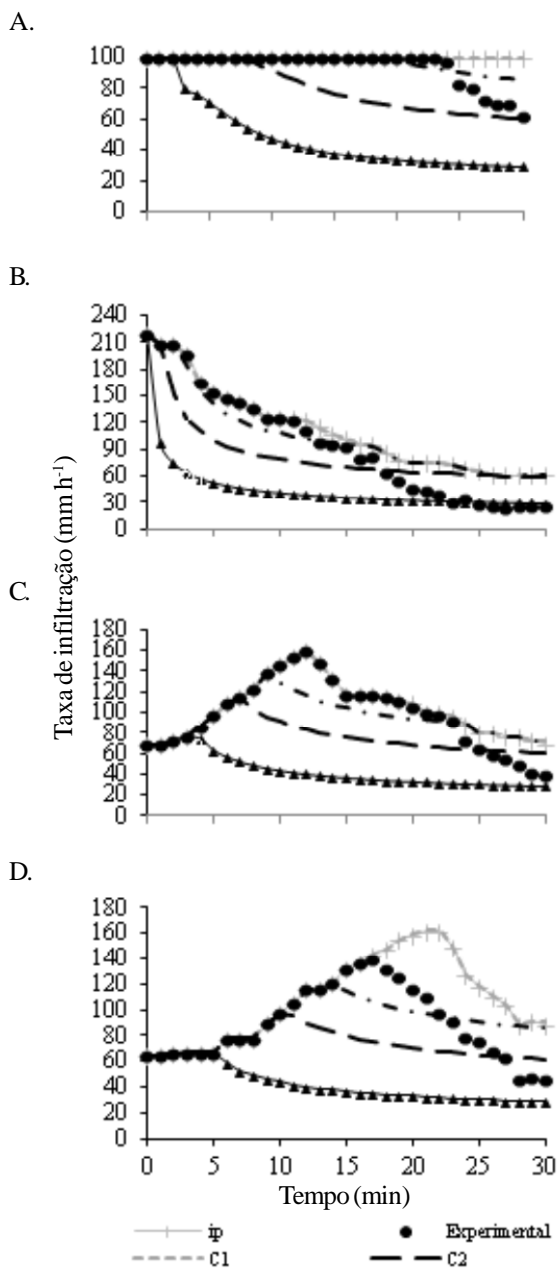
Fig 3. Taxa de infiltração medida e estimada pelo modelo de GAML usando-se diferentes combinações de seus parâmetros de entrada, 1ª aplicação, perfis de precipitação constante (A), exponencial decrescente (B), duplo exponencial adiantado (C) e atrasado (D)
