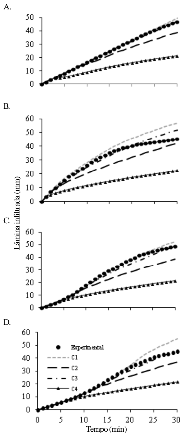
Figura 4. Lâmina infiltrada medida e estimada pelo modelo de GAML usando-se diferentes combinações de seus parâmetros de entrada, 1ª aplicação, perfis de precipitação constante (A), exponencial decrescente (B), duplo exponencial adiantado (C) e atrasado (D)
