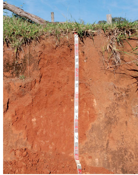
Figura 4.5 – Argissolo vermelho (PV) desenvolvido em relevo suave ondulado e ondulado (Ariquemes). Fonte: Ari Dêlcio Cavedon.
