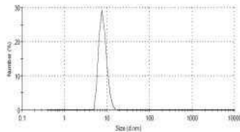
Fig.1: Distribuição do tamanho médio das partículas pela técnica de espalhamento dinâmico de luz.
