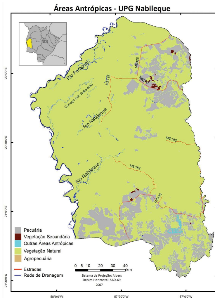
Figura 2 - Fitofisionomias mapeadas na UPG do Nabileque, Estado de Mato Grosso do Sul, escala 1:100.000, ano 2007.
