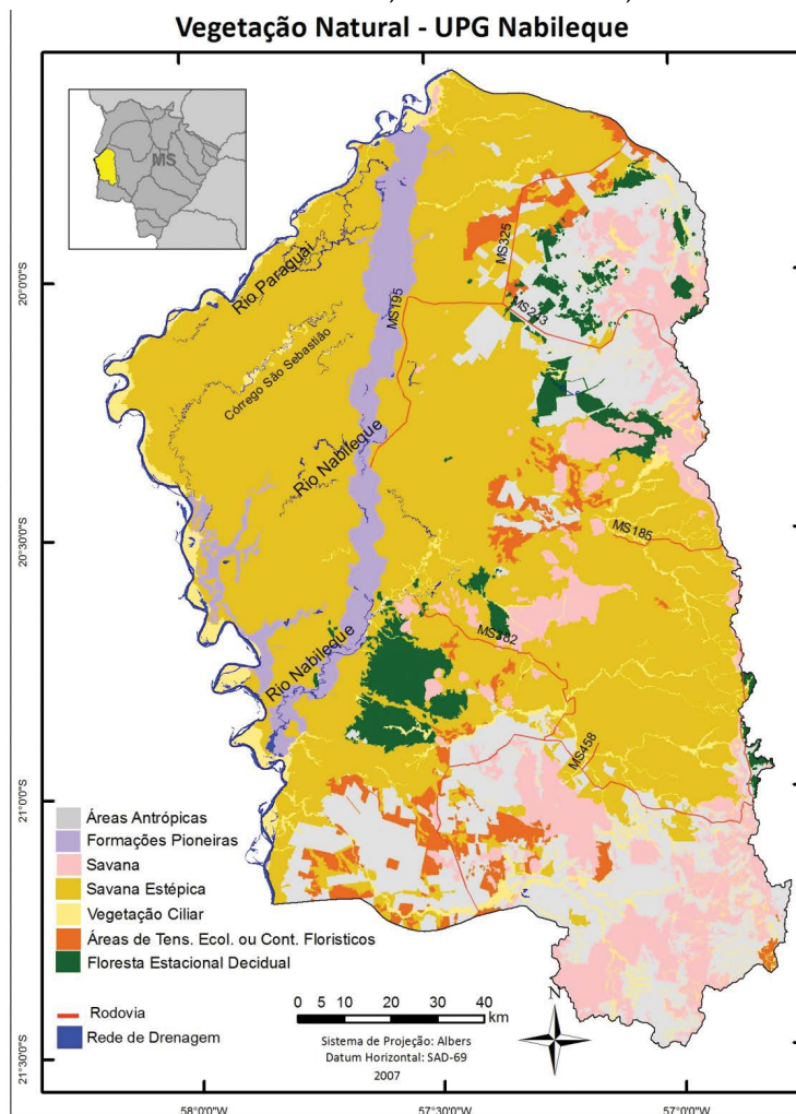
Figura 1 - Mapa da UPG do Nabileque indicado o uso da terra e a vegetação natural, Estado de Mato Grosso do Sul, escala 1:100.000, ano 2007.
