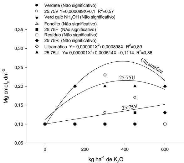
Figura 3: Disponibilidade de magnésio (Mg 2+ ) no solo em função dos tratamentos e das doses de K 2 O kg ha -1 após 45 dias de incubação
