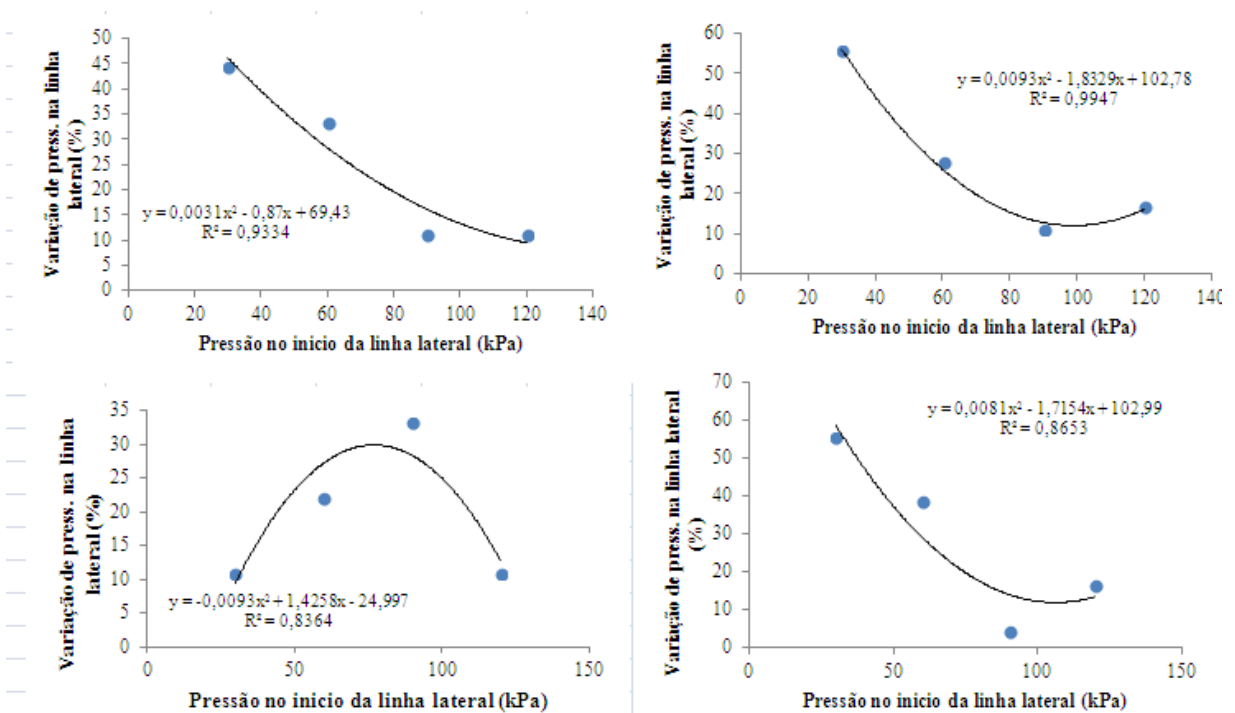
Figura 2. Percentagem de variação de pressão em função da pressão no início da linha lateral para (A) gotejador regulável de oito saídas, (B) gotejador tipo parafuso, (C) gotejador autocompensante e (D) microaspersor difusor.
