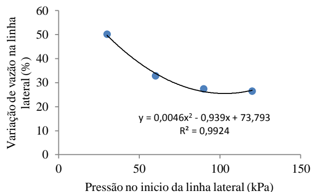
Figura 1. Percentagem de variação de vazão em função da pressão no início da linha lateral.
