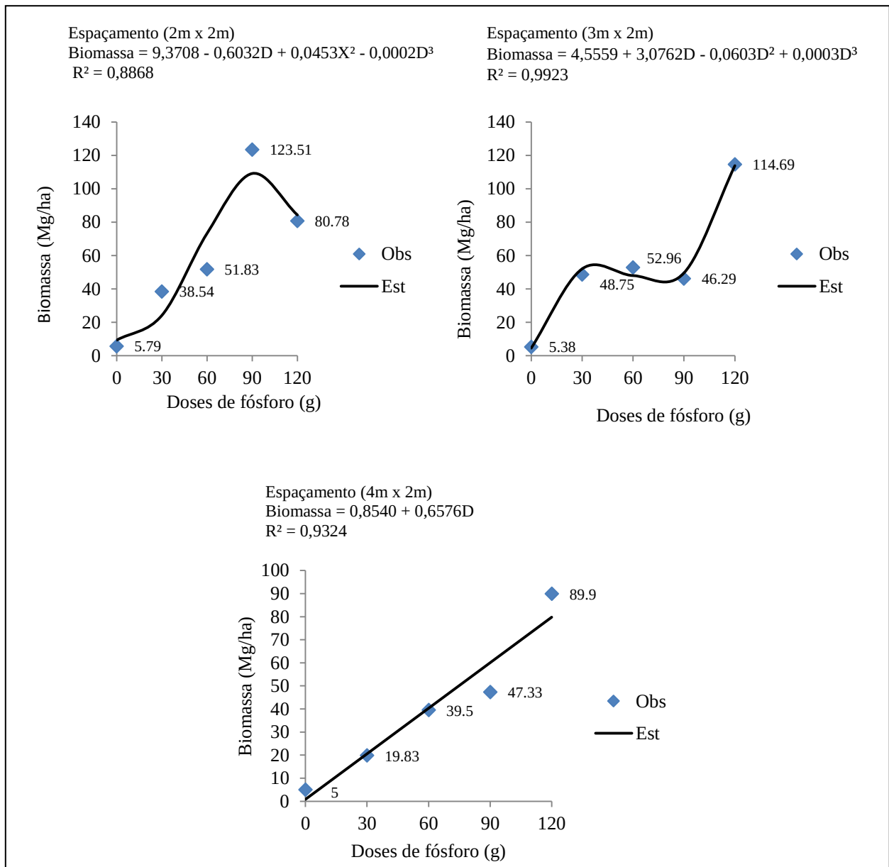
Figura 25 - Regressão da biomassa de E. urograndis em função das doses de fósforo por espaçamento. Legenda: Mg = megagrama (1Mg = 10^6 g); D = Doses de fósforo.
