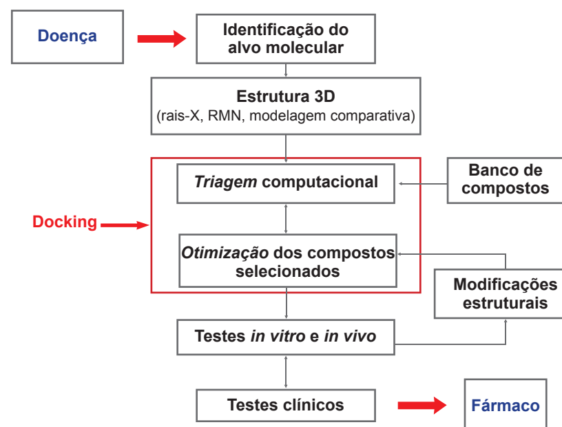
Figura 1. Fluxograma com as etapas básicas do desenho racional de fármacos baseado em estrutura.
