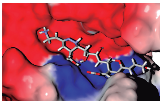
Figura 5. Ligante dh3211 posicionado no sítio-alvo da 1HG8 (PDB).
