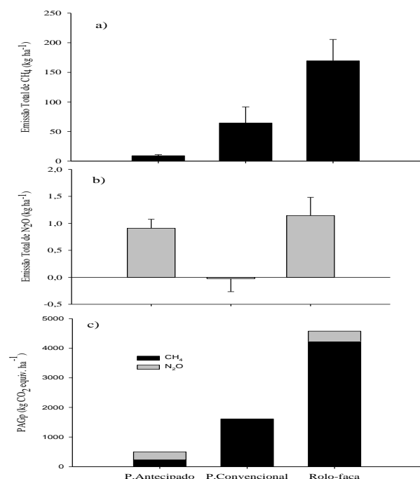
Figura 2. Emissão total de \text{CH}_4 (a), de \text{N}_2\text{O} (b) e o Potencial de Aquecimento Global parcial (c) em Planossolo durante o outono/inverno, sob distintos sistemas de preparo. Barras verticais representam o desvio padrão da média.
