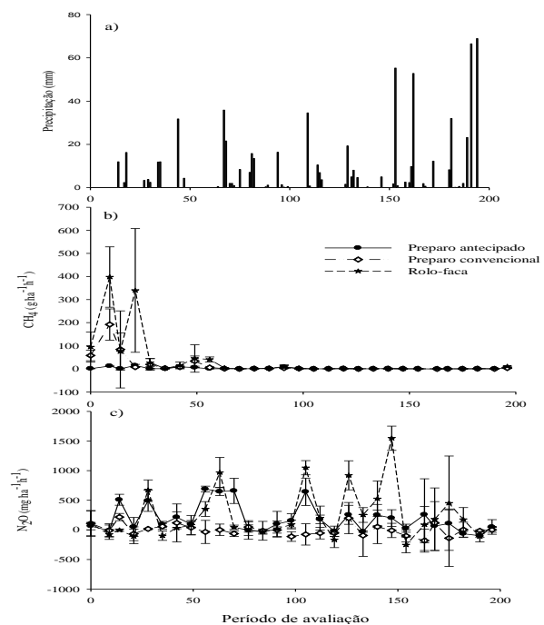
Figura 1. Precipitação pluviométrica (a) e fluxos de \text{CH}_4 (b) e de \text{N}_2\text{O} (c) em Planossolo durante o outono/inverno, sob distintos sistemas de preparo. Barras verticais representam o desvio padrão da média.
