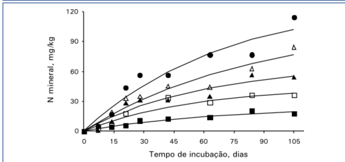
FIGURA 1 - PRODUÇÃO ACUMULADA OBSERVADA (PONTOS) E ESTIMADA (LINHAS) DE N MINERAL EM LATOSSOLO INCUBADO DURANTE 105 DIAS COM LODO DE ESGOTO COLETADO EM 1999 NA ESTAÇÃO DE TRATAMENTO DE ESGOTO DE FRANCA/SP (■: TESTEMUNHA (SEM LODO); □: 3; ▲: 6; △: 12 E ●: 24 T/HA DE LODO DE ESGOTO)
