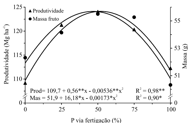
Figura 3. Produtividade e massa de frutos comerciais, conforme a percentagem de P aplicada via fertirrigação ao tomateiro, no experimento 2.
