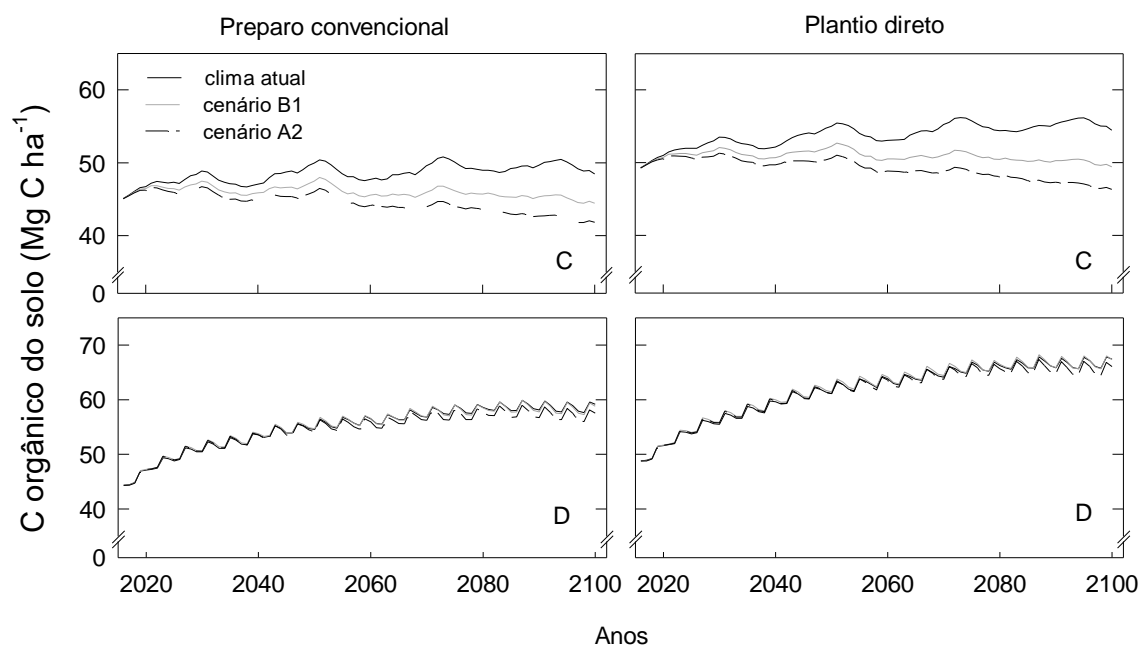
Figura 27. C orgânico do solo simulado sob cenários alternativos de manejo e de clima. C – trigo-soja-ervilhaca-sorgo-ervilhaca-sorgo; D – 2 anos Tifton-trigo-soja-trigo/soja.
