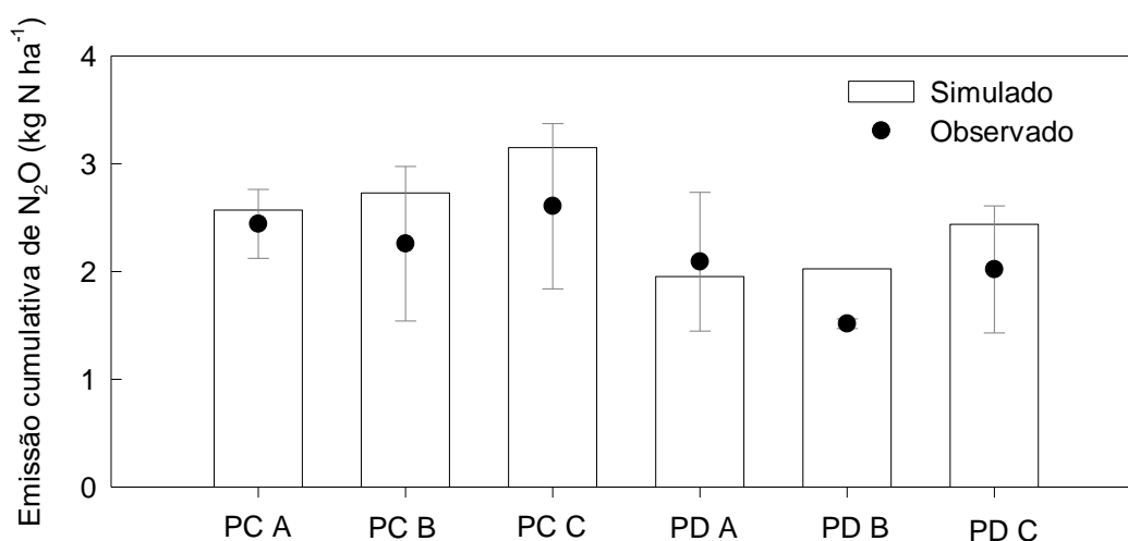
Figura 20. Emissões cumulativas de N_2O simuladas e observadas \pm desvio padrão em preparo convencional (PC) e plantio direto (PD) durante dois anos de avaliação. A – trigo-soja-trigo-soja; B – trigo-soja-ervilhaca-sorgo; C – ervilhaca-sorgo-trigo-soja.
