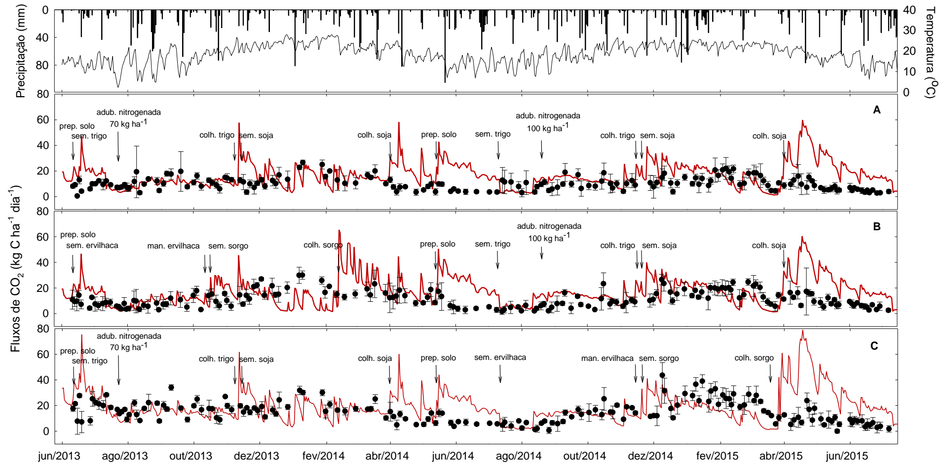
Figura 15. Fluxos de CO 2 simulados e medidos \pm desvio padrão durante o período de avaliação nos sistemas de culturas em preparo convencional. A – trigo-soja-trigo-soja; B – trigo-soja-ervilhaca-sorgo; C – ervilhaca-sorgo-trigo-soja.
