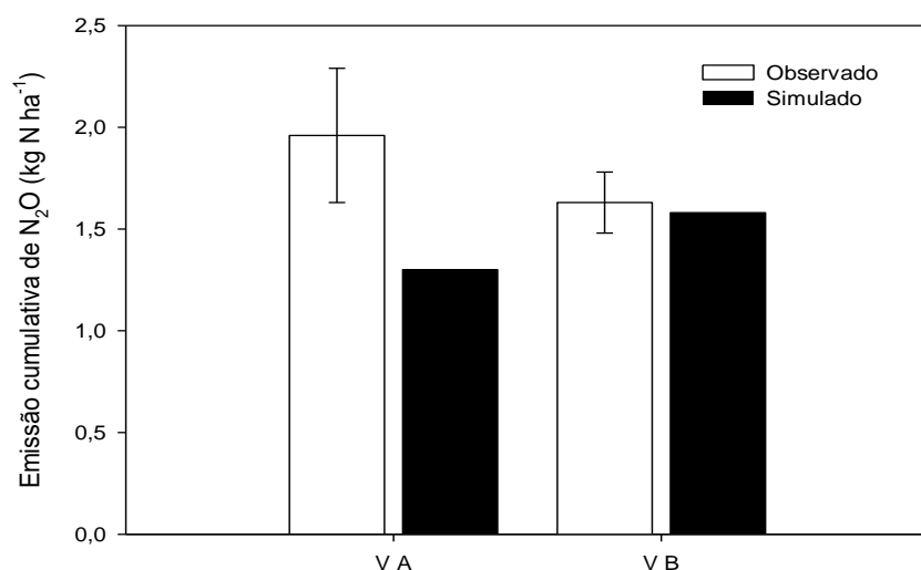
Figura 25. Emissão cumulativa de N 2 O simuladas e observadas \pm desvio padrão em dois sistemas de culturas do experimento 2 na etapa de validação do modelo. VA – trigo-soja; VB – trigo-soja-ervilhaca-sorgo-aveia-soja.
