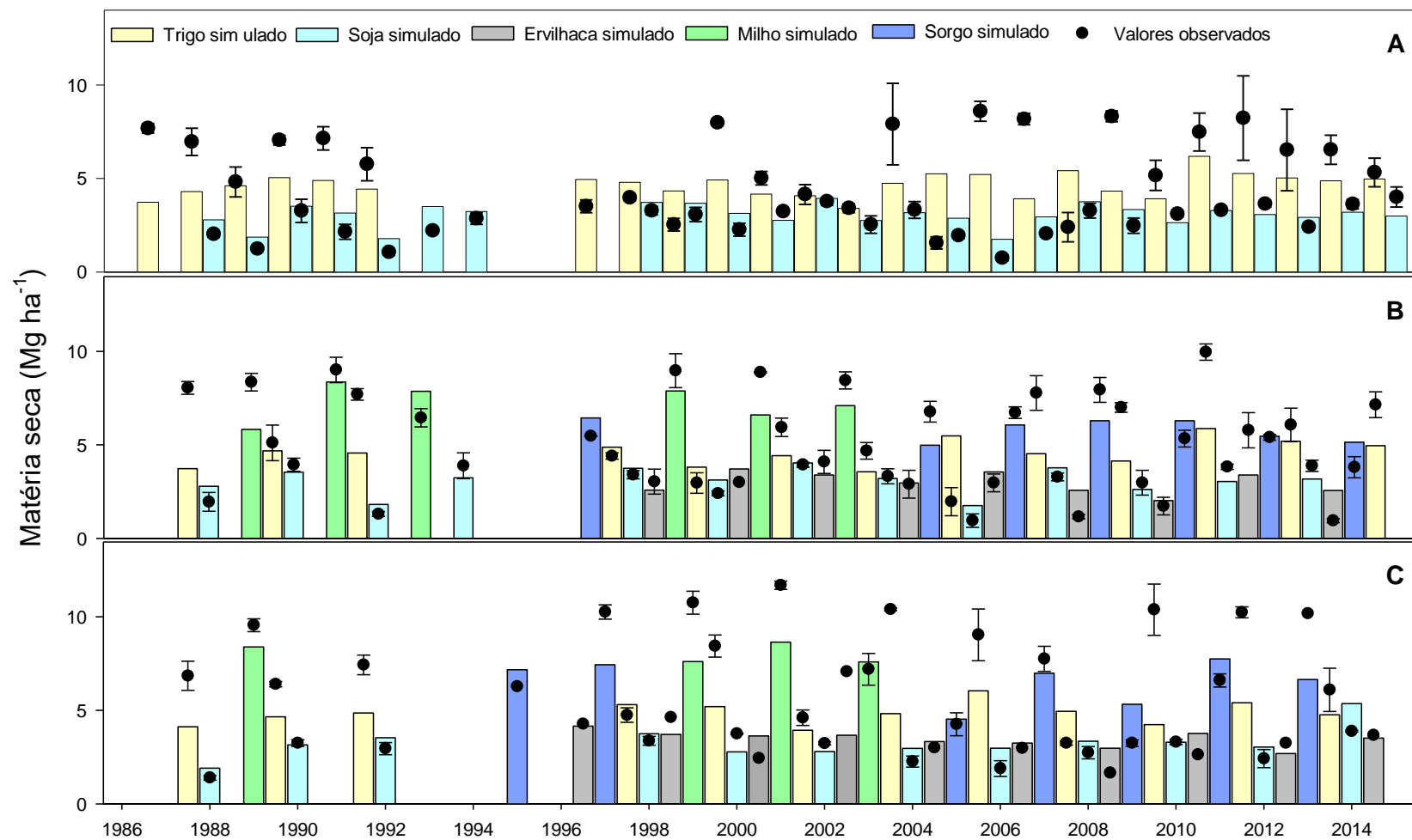
Figura 8. Produção anual de biomassa (parte aérea) simulada e observada \pm desvio padrão durante os 28 anos de plantio direto. A – trigo-soja; B – trigo-soja-ervilhaca-milho (sorgo); C – ervilhaca-milho (sorgo) –trigo-soja.
