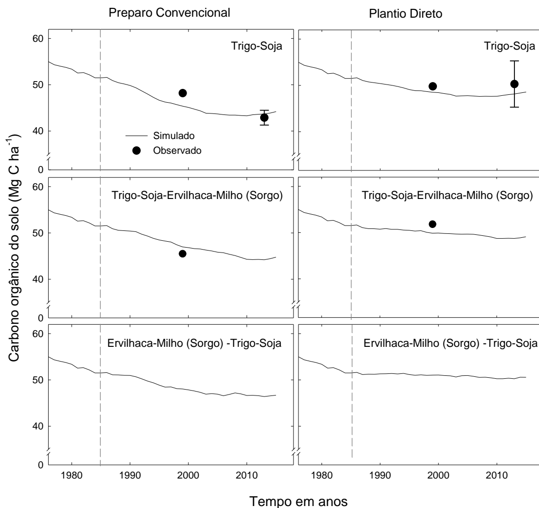
Figura 6. Carbono orgânico do solo simulado e observado \pm desvio padrão na camada 0-20 cm de solo durante o pré-experimento e período experimental em preparo convencional e plantio direto. O tracejado vertical indica o início do experimento.
