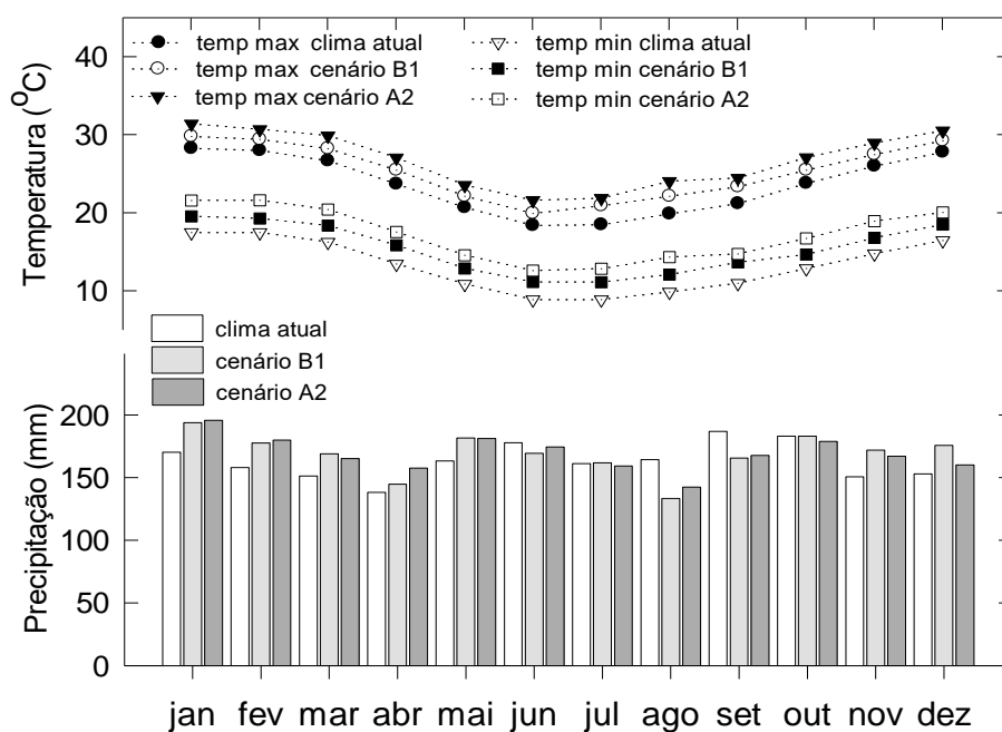
Figura 3. Alterações das temperaturas médias máximas e mínimas mensais e da distribuição da precipitação mensal sob os cenários climáticos atual, B1 e A2.
