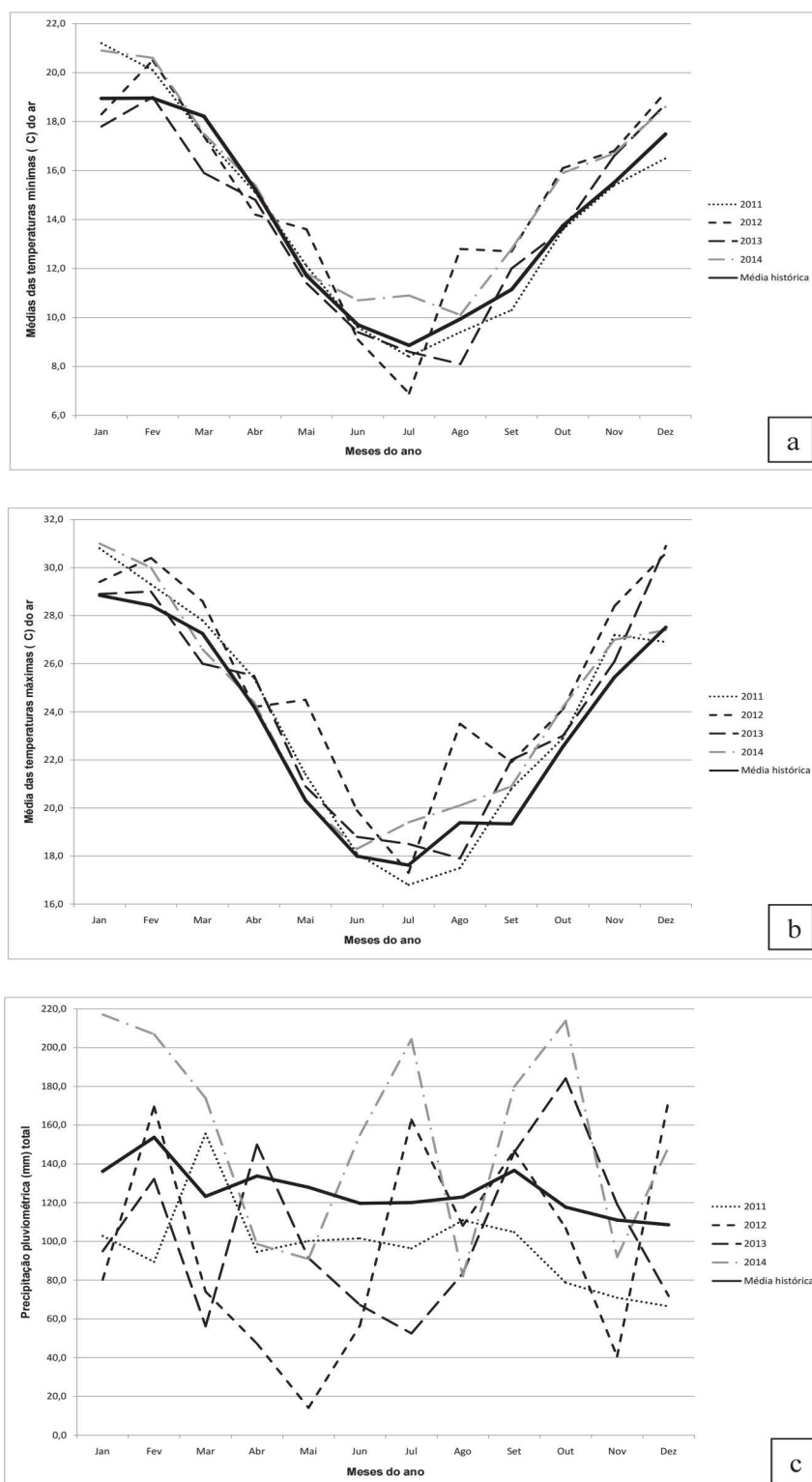
Figura 1 - Médias das temperaturas mínimas (a) e máximas (b) do ar e precipitação pluviométrica total (c), registradas na sede da Embrapa Clima Temperado durante a avaliação do experimento (2011-2014) e médias históricas (1984-2010). Fonte: http://www.cpact.embrapa.br/agromet/ .
