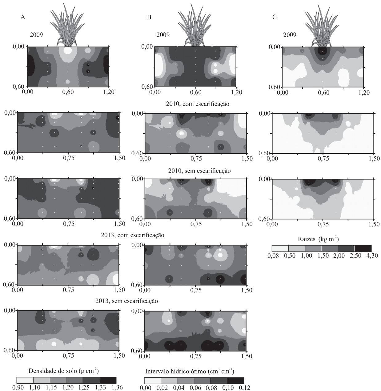
Figura 5. Distribuição espacial da densidade do solo (A), do intervalo hídrico ótimo (B) e da massa específica de raízes no perfil (C) de um Latossolo Vermelho acriférico típico, nas condições estudadas.
