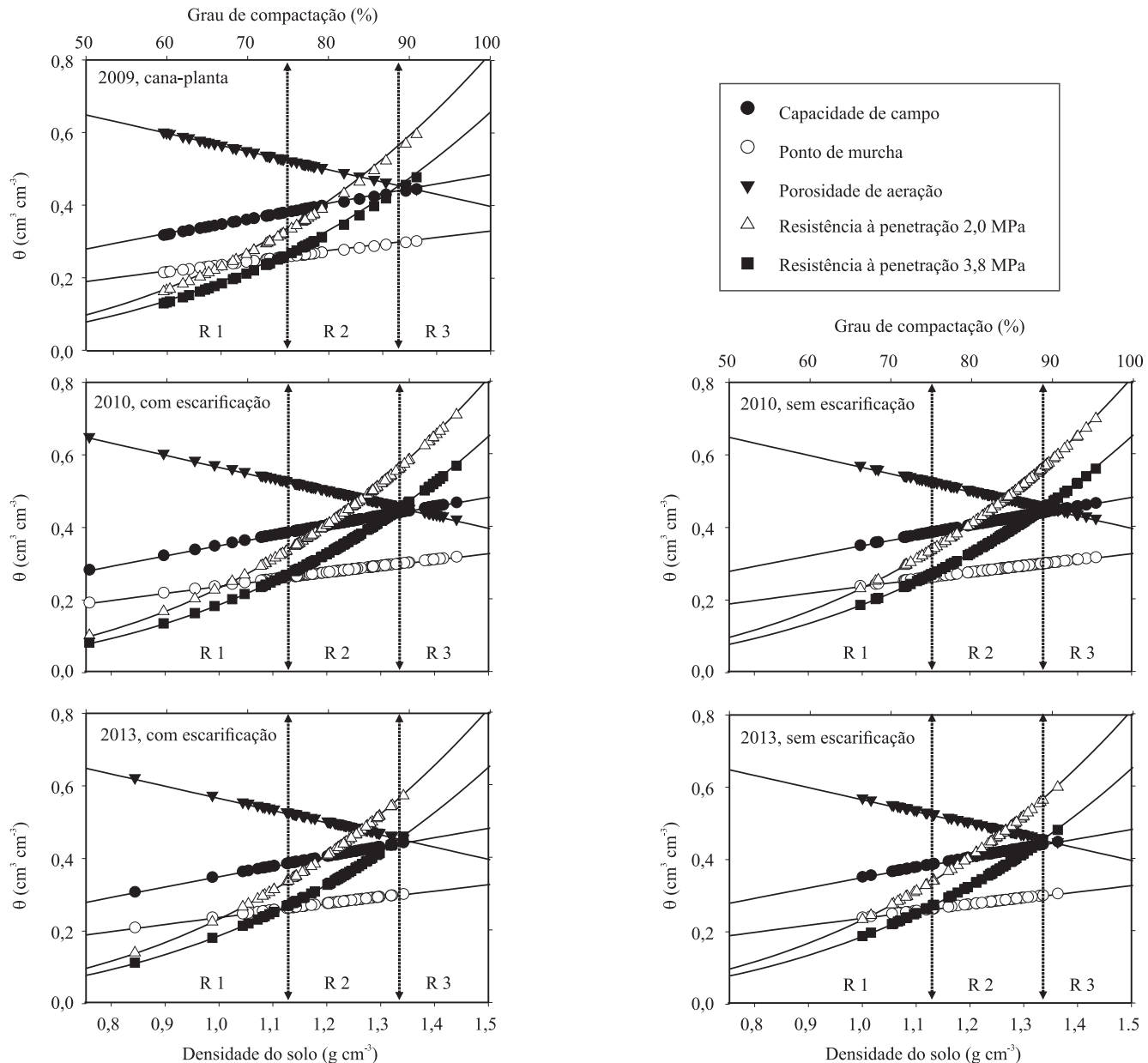
Figura 4. Diagramas de intervalo hídrico ótimo de Latosolo Vermelho acriférico típico, textura muito argilosa, nos anos de 2009; 2010 e 2013. As regiões R1, R2 e R3 correspondem, respectivamente, à região sem impedimentos físicos ao crescimento de raízes; às regiões com impedimentos e limitações ao crescimento radicular.
