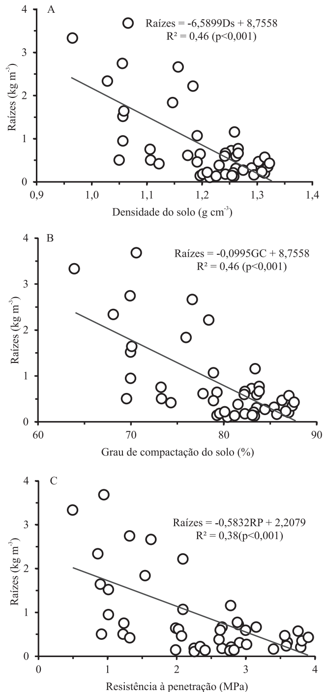
Figura 3. Relações da massa específica de raízes com: A, densidade do solo (Ds); B, grau de compactação do solo (GC); e C, resistência mecânica à penetração (RP) corrigida para teor de água equivalente à tensão mátrica de 6 kPa.
