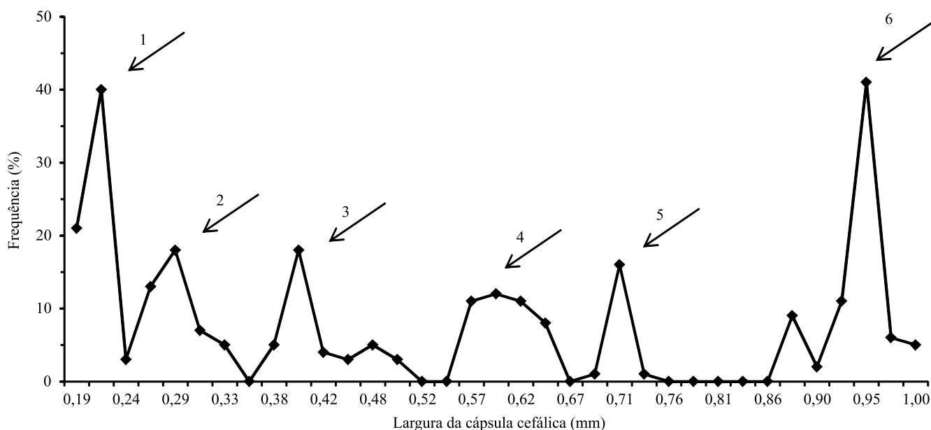
Figura 1. Distribuição de frequência das medidas de largura de cápsula cefálica de Strepsicrates smithiana em araçazeiro. As setas indicam o número de instares. Temperatura de 25 \pm 2^\circ\text{C} , umidade relativa de 70 \pm 20\% e fotófase de 12 horas.
