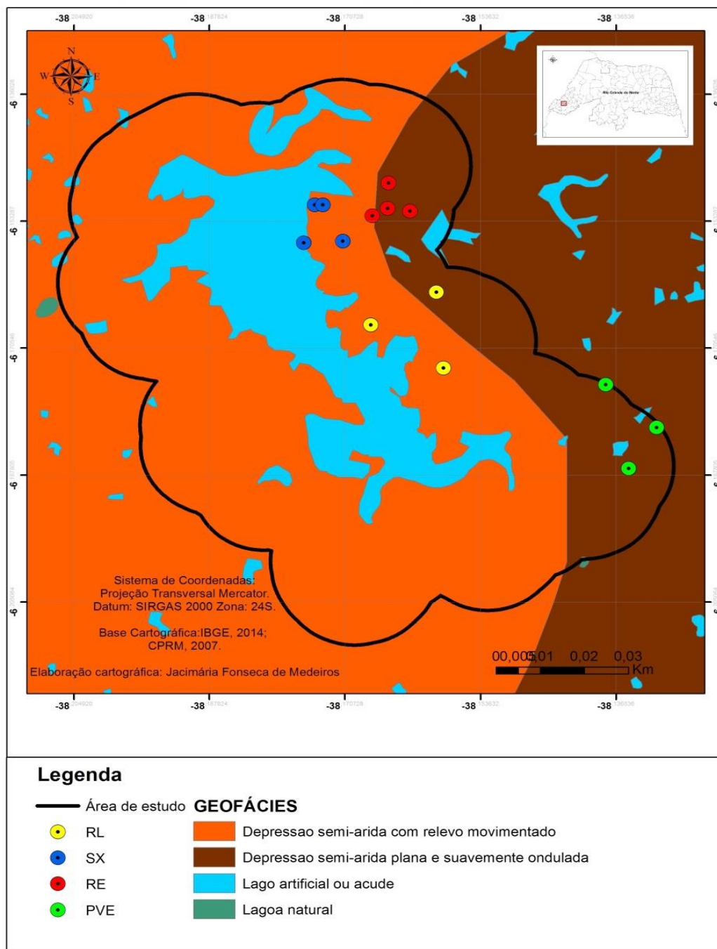
Figura 2: Mapa dos Geofácies e da localização dos solos identificados na área de estudo
