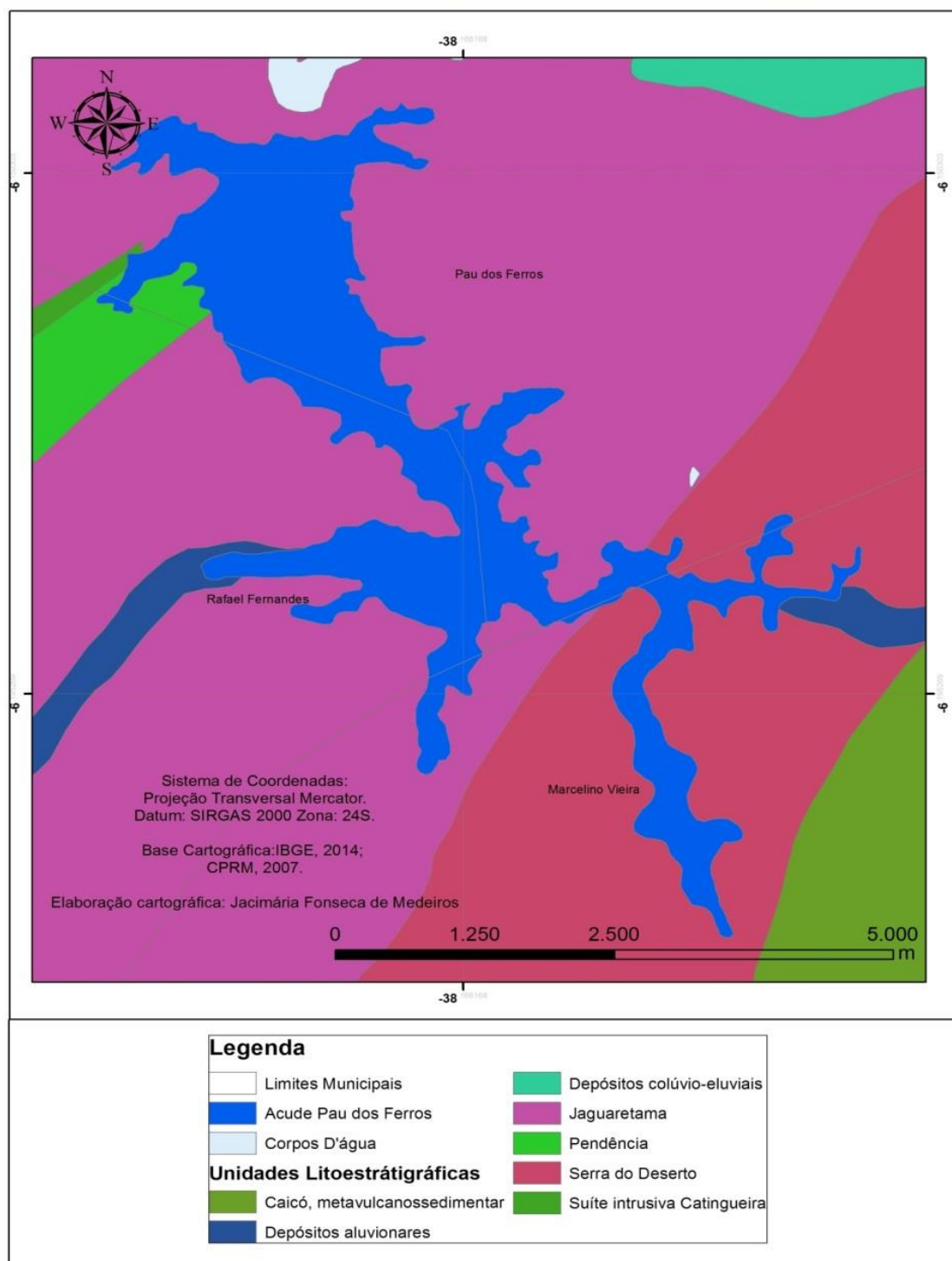
Figura 01- Geologia predominante na área de estudo
