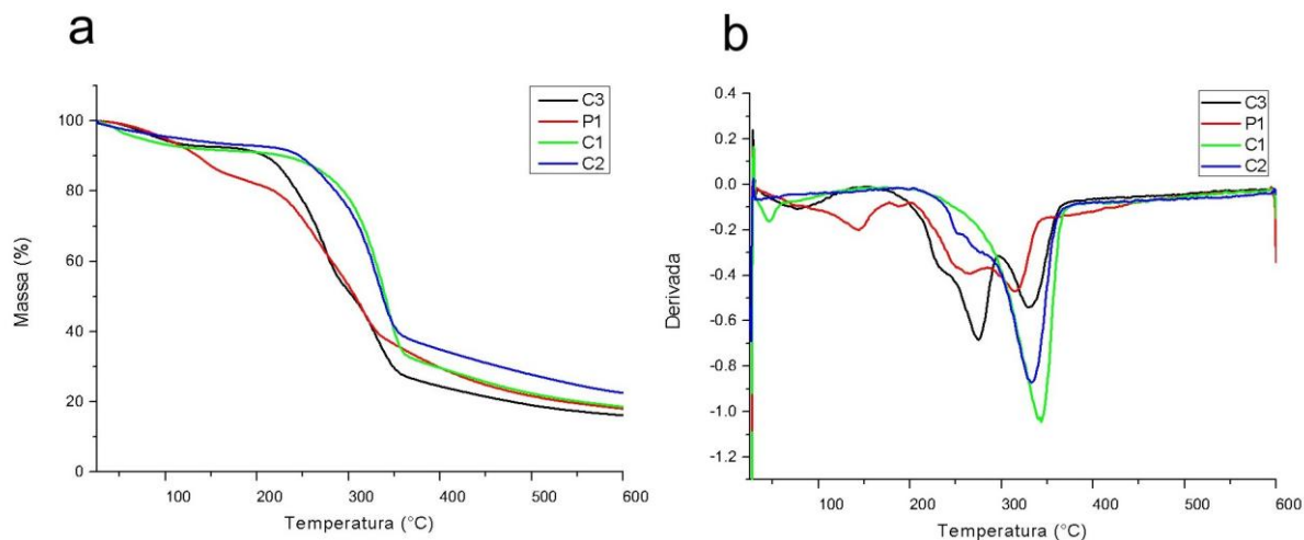
Figura 2 – Perfil termogravimétrico dos filmes
