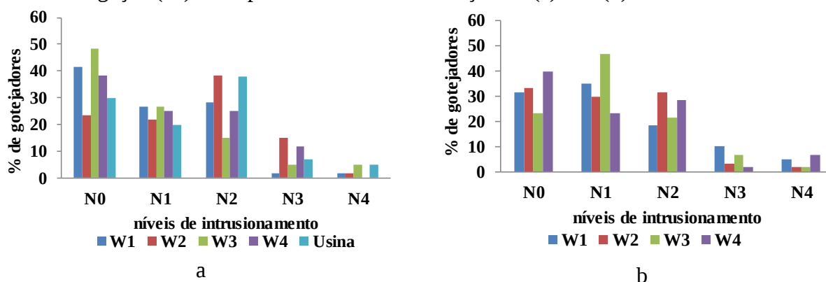
Figura 2. Percentual de gotejadores, por nível de intrusão da raiz (N), em função dos níveis de irrigação (W) e das profundidades de instalação P1 (a) e P2(b).
