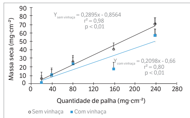
Figura 3. Massa seca remanescente da palha de cana-de-açúcar em função das quantidades de palha (0; 20; 40; 80; 160 e 240 mg·cm -2 ) e da aplicação ou não de vinhaça. Barras verticais representam a diferença mínima significativa pelo teste de Tukey ( p \leq 0,05 ) entre as quantidades médias de massa seca remanescente nos tratamentos com e sem aplicação de vinhaça.
