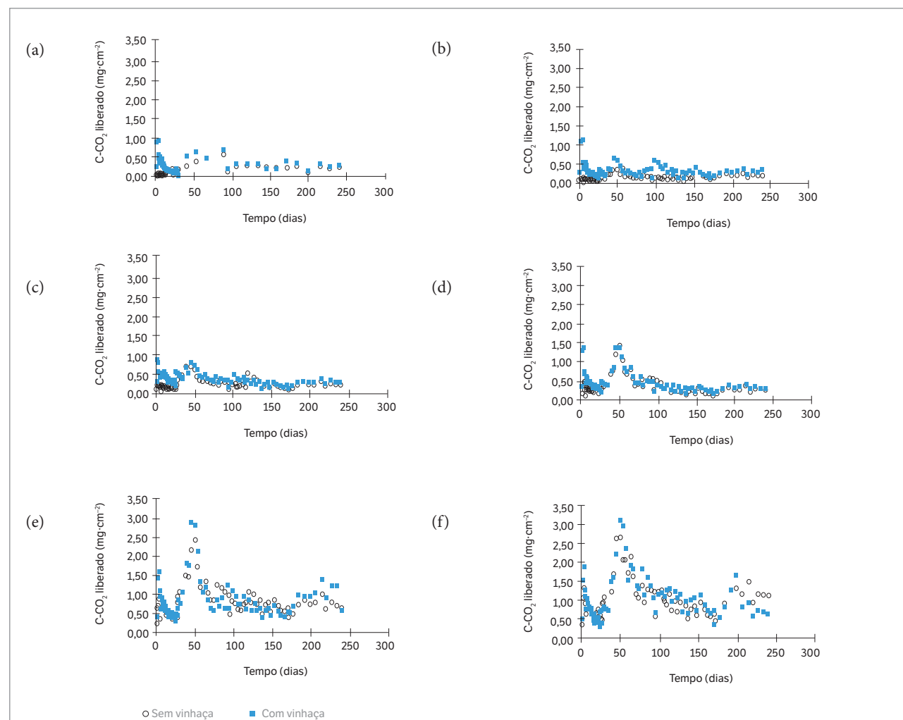
Figura 1. Carbono liberado na forma \text{CO}_2 ( C\text{-CO}_2 ) em função do tempo de incubação e com ou sem aplicação de vinhaça. (a) 0 \text{t}\cdot\text{ha}^{-1} de palha; (b) 2 \text{t}\cdot\text{ha}^{-1} de palha (20 \text{mg}\cdot\text{cm}^{-2} ); (c) 4 \text{t}\cdot\text{ha}^{-1} de palha (40 \text{mg}\cdot\text{cm}^{-2} ); (d) 8 \text{t}\cdot\text{ha}^{-1} de palha (80 \text{mg}\cdot\text{cm}^{-2} ); (e) 16 \text{t}\cdot\text{ha}^{-1} de palha (160 \text{mg}\cdot\text{cm}^{-2} ); (f) 24 \text{t}\cdot\text{ha}^{-1} de palha (240 \text{mg}\cdot\text{cm}^{-2} ).
