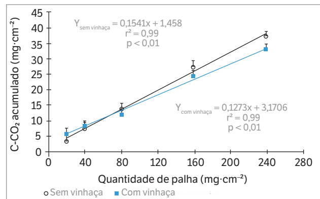
Figura 2. Carbono acumulado na forma de CO 2 (C-CO 2 ), em função das quantidades de palha de cana-de-açúcar (0; 20; 40; 80; 160 e 240 mg·cm -2 ) e o efeito com e sem aplicação de vinhaça. Barras verticais representam a diferença mínima significativa entre C-CO 2 acumulado dentro de cada tempo de avaliação.
