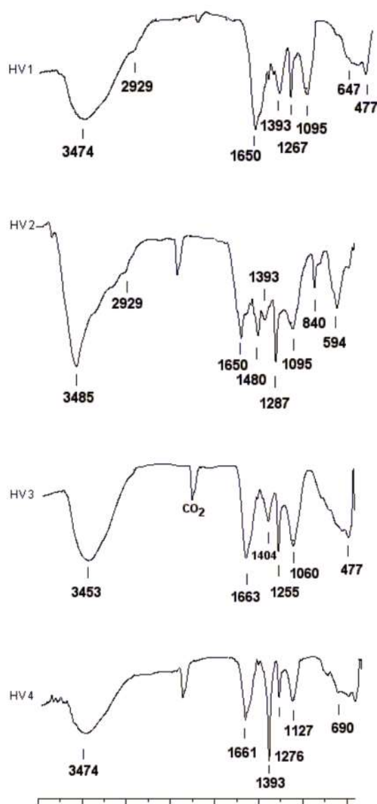
Figura 1. Espectros na região de infravermelho com transformada de Fourier (em cm -1 ) dos humatos extraídos de vermicomposto de esterco de curral (HV1), de esterco de curral + bagaço de cana-de-açúcar (HV2), de esterco de curral + folhas de leguminosas (HV3) e de esterco de curral + bagaço de cana-de-açúcar + folhas de leguminosas (HV4)
