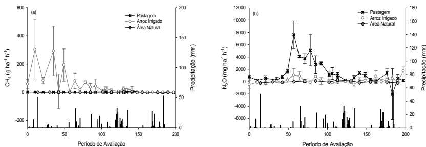
Figura 1. Precipitação pluviométrica e fluxos de CH_4 (a) e de N_2O (b) no outono/inverno, em Planossolo cultivado com arroz irrigado e pastagens no verão, comparativamente à área natural. Barras verticais representam o desvio padrão da média. Embrapa Clima Temperado. Capão do Leão, RS. 2016.
