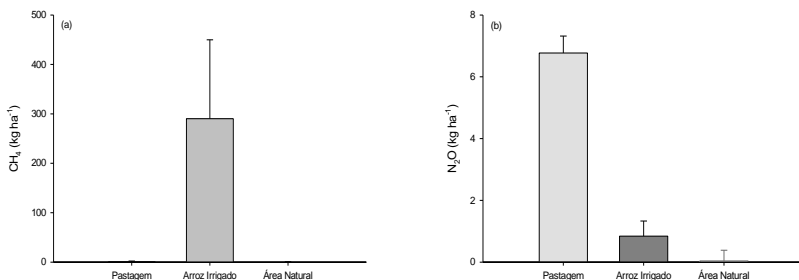
Figura 2. Emissões totais de CH_4 (a) e de N_2O (b) no outono/inverno, em Planossolo cultivado com arroz irrigado e pastagens no verão, comparativamente à área natural. Barras verticais representam o desvio padrão da média. Embrapa Clima Temperado. Capão do Leão, RS. 2016.
