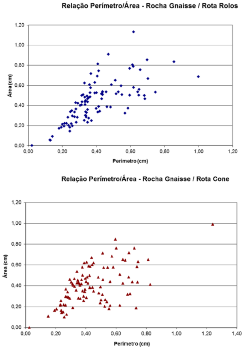
Figura 9 – Retas de regressão linear aplicada aos dados brutos de perímetro e área de grãos da rocha Gnaiss produzidos em duas rotas de cominuição (Carneiro, 2016)
