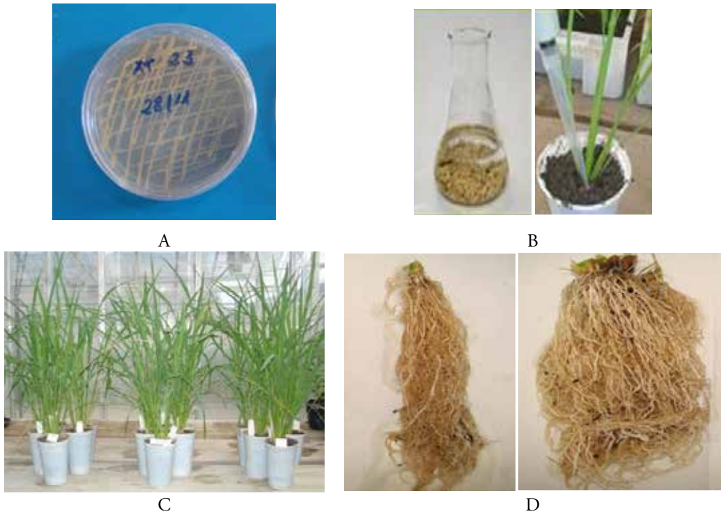
Figura 7 – Etapas dos testes in vivo com micro-organismos isolados da rocha folhelho pirobetuminoso (xisto) na cultura do arroz irrigado: isolamento do micro-organismo de interesse (a), introdução do isolado na semente ou no solo (b), avaliação do desenvolvimento da parte aérea das plantas inoculadas (c) e avaliação das raízes das plantas testemunha e inoculada com o micro-organismo de interesse, respectivamente (d). Embrapa Clima Temperado, 2013. Fotos: Cesar B. Gomes.
