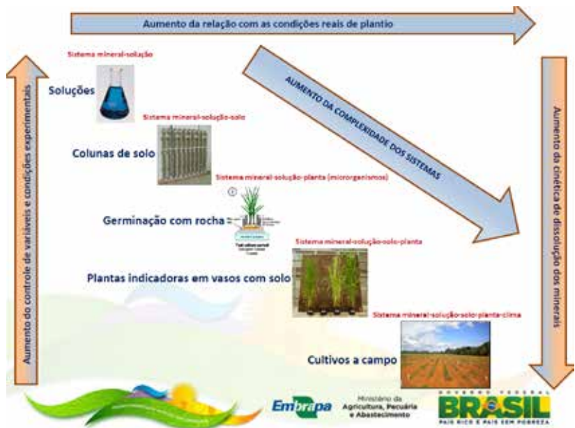
Figura 5 – Esquema conceitual das relações entre os tipos de experimentos e a complexidade dos sistemas nos estudos de remineralização (Martins, 2013).
