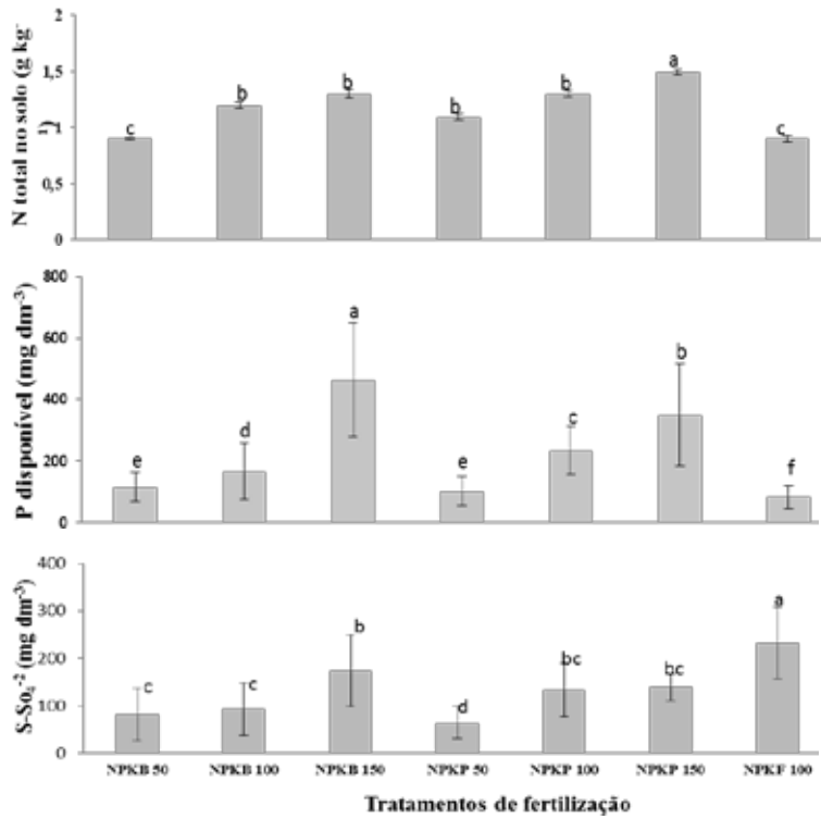
Figura 8 – N total, P disponível e \text{SO}_4^{2-} solúvel em solo da Zona da Mata de Pernambuco cultivado com pimentão com diferentes doses de biofertilizante, fertilizante mineral e húmus de minhoca.
