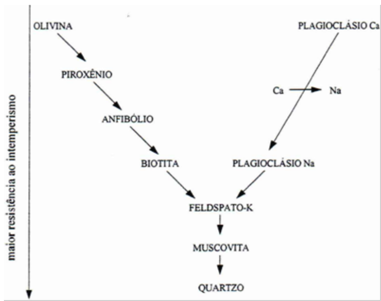
Figura 6 – Sequência de resistência dos minerais ao intemperismo (Goldish, 1938)
