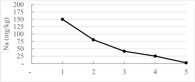
Figura 7 – Concentração de Na e Ca na suspensão da fração Areia Fina do RM em água, em tubos de ensaio, em cada uma de cinco extrações consecutivas (adaptado de Silva,2016)
