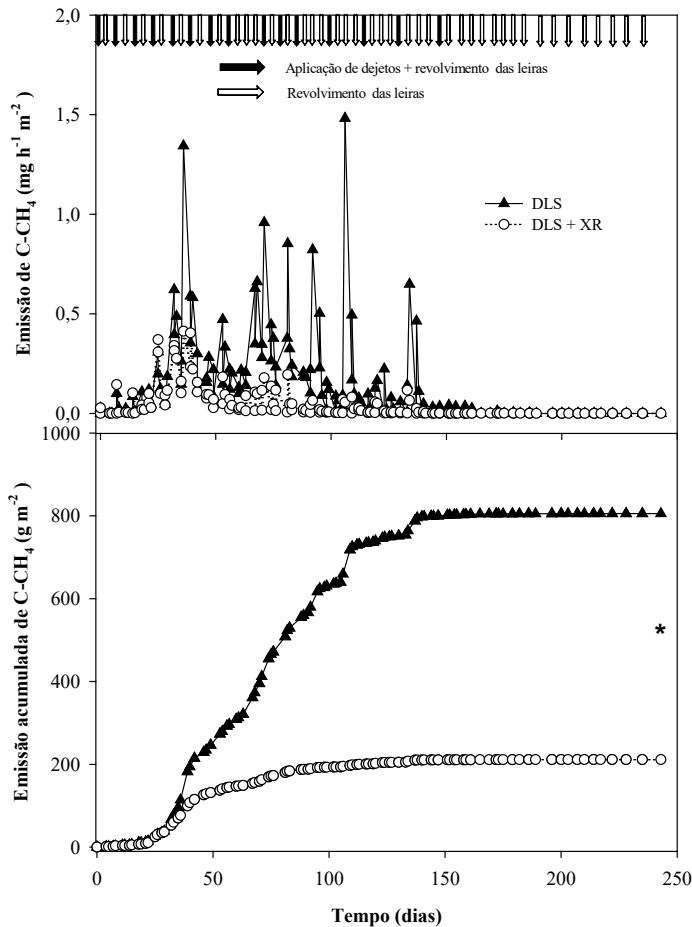
Figura 6 – Fluxos e emissões acumuladas de C-CH 4 em compostagem automatizada de dejetos líquidos de suínos (DLS), com e sem a adição de xisto retortado (XR). * = diferença mínima significativa pelo teste t (5%).
