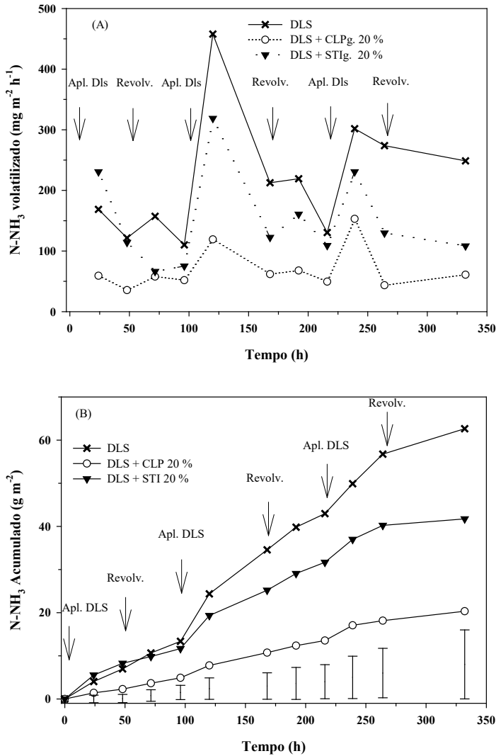
Figura 2 – Fluxos de \text{N-NH}_3 (a), emissão acumulada de \text{N-NH}_3 (b) em compostagem de dejetos líquidos de suínos (DLS) com e sem adição das zeólitas clinoptilolita e estilbita na dose de 20% (massa/massa). As barras verticais (b) representam a diferença mínima significativa pelo teste LSD (5 %). As flechas, (Figuras a, b), indicam os momentos de aplicação (Apl.) dos DLS e de revolvimento (Revolv.) da massa de compostagem.
