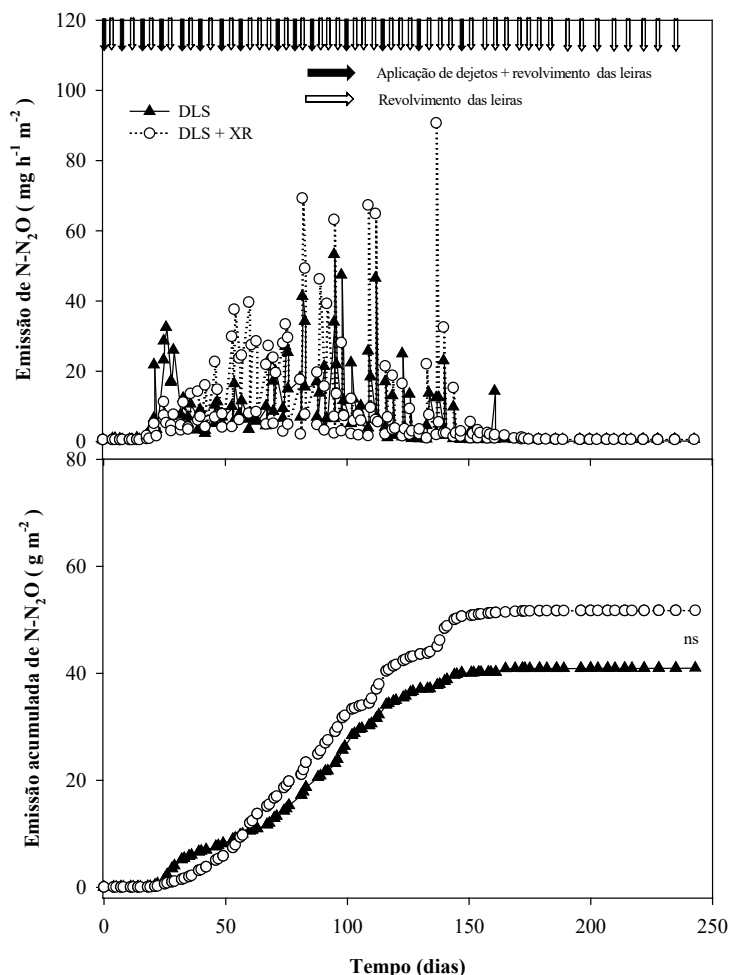
Figura 5 – Fluxos e emissões acumuladas de N-N_2O em compostagem automatizada de dejetos líquidos de suínos, onde DLS (dejetos líquidos de suínos) e XR (xisto retornado). ns= diferença não significativa pelo teste t (5%).
