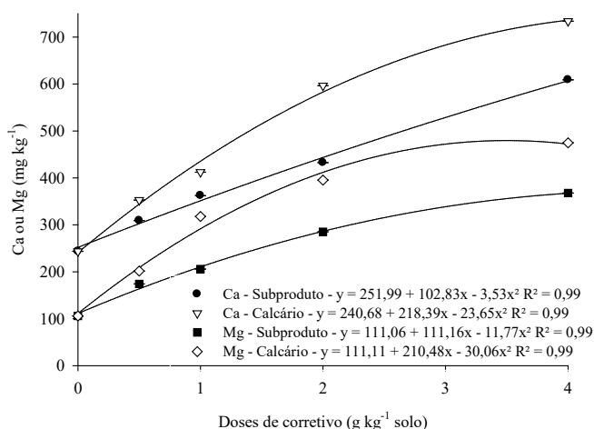
Figura 2 – Teores de Ca e Mg no solo submetidos a aplicação de calcário e subproduto.
