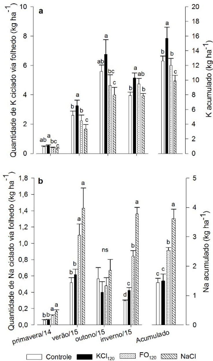
Figura 1 – Ciclagem de K (a) e Na (b) via produção de folheto em plantio de eucalipto fertilizado com KCl, NaCl e fonolito. Barras acima das colunas representam o erro padrão da média. ns - diferença não significativa (teste F, \alpha=0,1 ). Colunas seguidas pela mesma letra minúscula não diferem entre si pelo teste LSD ( \alpha=0,05 )
