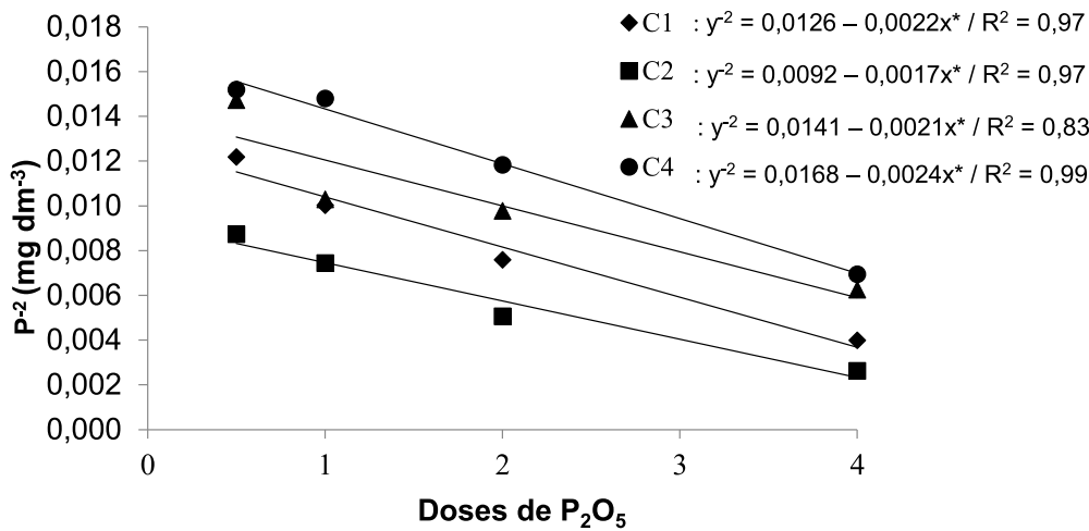
Figura 1 – Curvas respostas de fósforo (P, variável transformada y^{-2} ) disponível no solo em função de doses de P_2O_5 (0,5; 1,0; 2,0; e 4,0 vezes a recomendada) após quatro coletas (C1, C2, C3 e C4).
