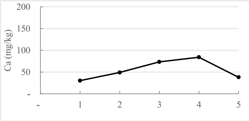
Figura 8 – Variação no Na e Ca trocáveis em amostras coletadas no solo remineralizado, em experimento de campo (adaptado de Silva,2016).
