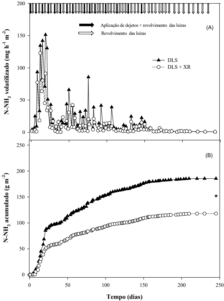
Figura 3 – Fluxo (A) e emissão acumulada (B) de amônia em compostagem automatizada de dejetos líquidos de suínos, onde DLS (dejetos líquidos de suínos) e XR (xisto retornado). Barra de erro indica a diferença mínima significativa pelo teste t (5%).
