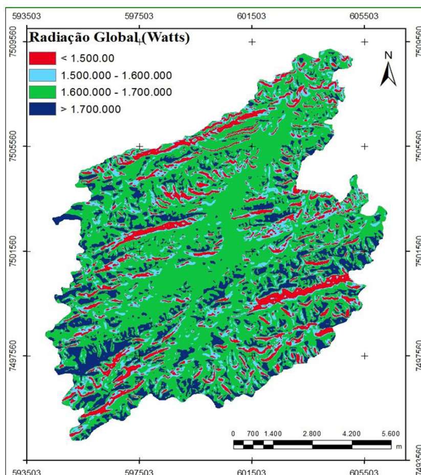
Figura 4. Mapa de radiação solar global da sub-bacia ribeirão Cachimbal, Pinheiral-RJ.
