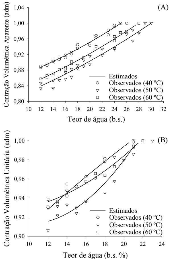
Figura 3. Valores observados e estimados da contração volumétrica aparente (A) e unitária (B) de grãos de soja da variedade NS7901RR pelo modelo Polinomial em função do teor de água para as temperaturas estudadas.
