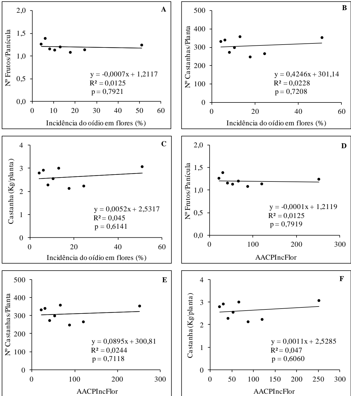
Figura 2 - Relação entre a incidência do oídio em flores (IncFlor) de cajueiro ano BRS 189 e o número de frutos produzidos/panícula (A), o número de castanhas produzidas/planta (B), e a produção (Kg) de castanhas/planta (C); Relação entre a área abaixo da curva da incidência do oídio em flores (AACPIncFlor) de cajueiro e o número de frutos produzidos/panícula (D), o número de castanhas produzidas/planta (E), e a produção (Kg) de castanhas/planta (F).
