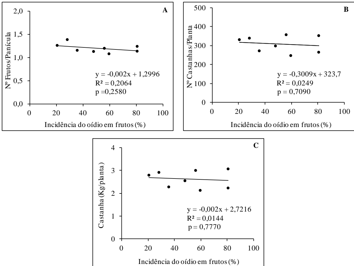
Figura 3 - Relação entre a incidência do oídio em frutos (IncFruto) de cajueiro anão BRS 189 (castanha+pedúnculo) e o número de frutos produzidos/panícula (A), o número de castanhas produzidas/planta (B), e a produção (Kg) de castanhas/planta (C).
