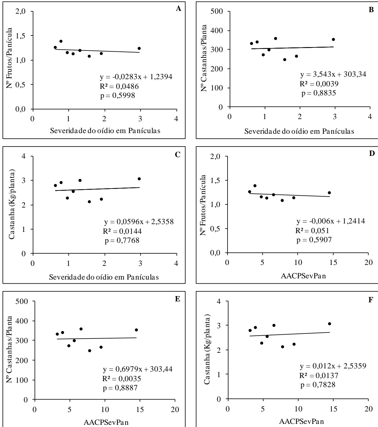
Figura 1 - Relação entre a severidade do oídio em panículas (SevPan) de cajueiro anão BRS 189 e o número de frutos produzidos por panícula (A), o número de castanhas produzidas por planta (B), e a produção (Kg) de castanhas/planta (C); Relação entre a área abaixo da curva de severidade do oídio em panículas (AACPSevPan) de cajueiro e o número de frutos produzidos/panícula (D), o número de castanhas produzidas/planta (E), e a produção (Kg) de castanhas/planta (F).
