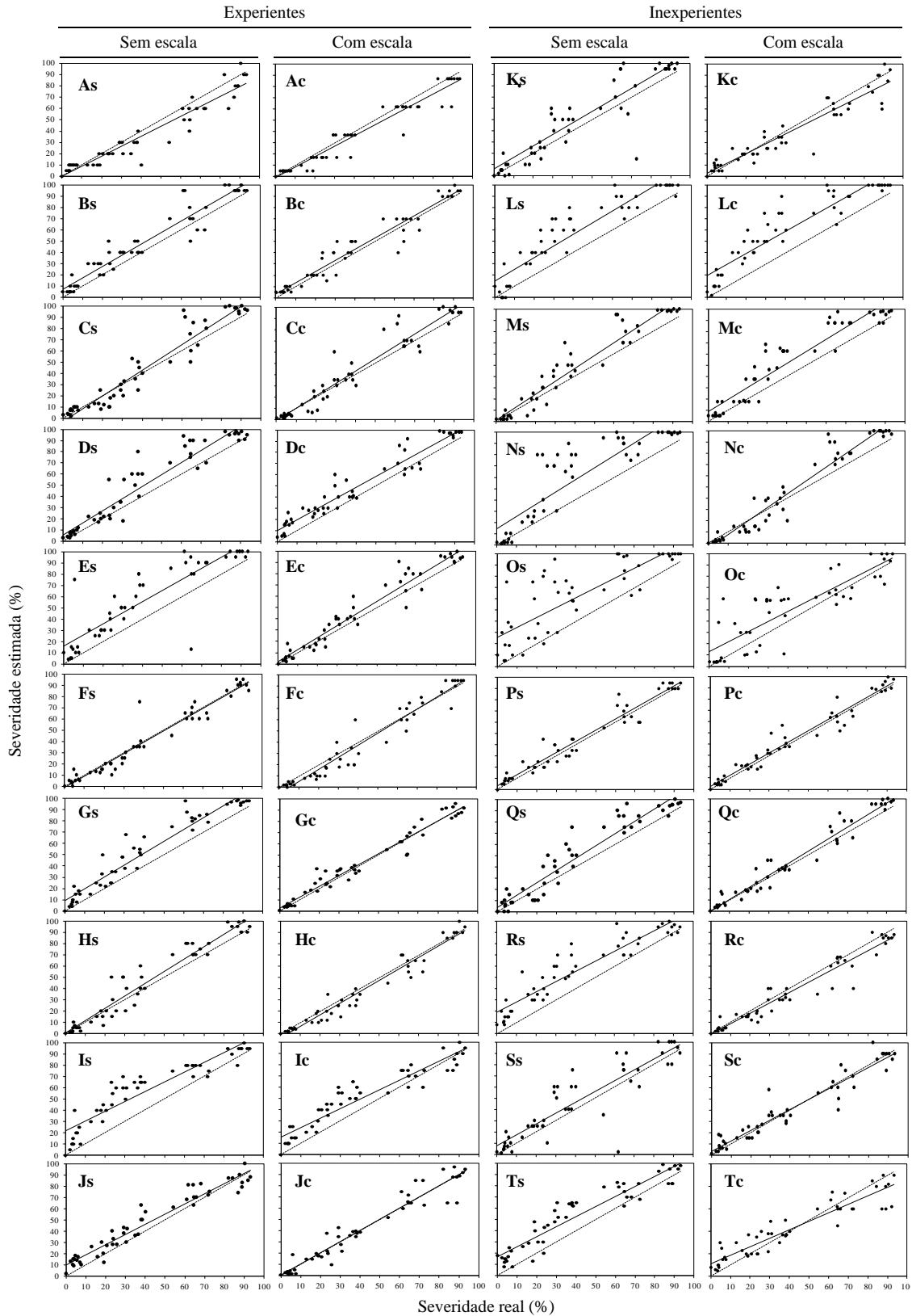
Figura 2 - Relação entre severidade real (%) e severidade estimada (%) (pontos cheios) para o oídio ( Pseudoidium anacardii ) em castanhas de cajueiro ( Anacardium occidentale ) por vinte avaliadores, sendo dez com experiência [sem (As, Bs, Cs, Ds, Es, Fs, Gs, Hs, Is, Js) e com (Ac, Bc, Cc, Dc, Ec, Fc, Gc, Hc, Ic, Jc) o uso da escala proposta] e dez sem experiência [sem (Ks, Ls, Ms, Ns, Os, Ps, Qs, Rs, Ss, Ts) e com (Kc, Lc, Mc, Nc, Oc, Pc, Qc, Rc, Sc, Tc) o uso da escala proposta]. A linha pontilhada, traçada pelo uso dos valores de severidade reais, representa a situação ideal.
