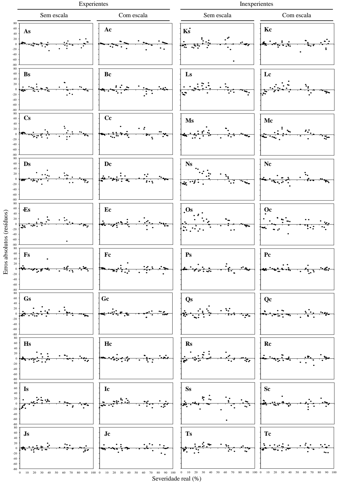
Figura 3 - Erros absolutos (severidade real menos severidade estimada) das estimativas da severidade do para o oídio ( Pseudoidium anacardii ) em castanhas de cajueiro ( Anacardium occidentale ) por vinte avaliadores, sendo dez com experiência [sem (As, Bs, Cs, Ds, Es, Fs, Gs, Hs, Is, Js) e com (Ac, Bc, Cc, Dc, Ec, Fc, Gc, Hc, Ic, Jc) o uso da escala proposta] e dez sem experiência [sem (Ks, Ls, Ms, Ns, Os, Ps, Qs, Rs, Ss, Ts) e com (Kc, Lc, Mc, Nc, Oc, Pc, Qc, Rc, Sc, Tc) o uso da escala proposta].
