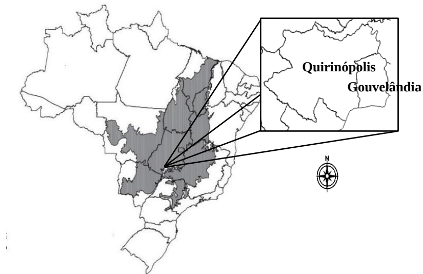
Figura 1. Localização dos municípios de Quirinópolis e Gouvelândia e a área de Cerrado (em cinza) no Brasil (SANO et al, 2007).
