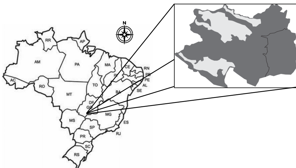
Figura 1. Localização dos municípios de Quirinópolis e Gouvelândia, Estado de Goiás, Brasil. Nas áreas em cinza escuro predominam Latossolos Vermelhos e em áreas em cinza claro predominam Argissolos Vermelho-Amarelo. Fonte: adaptado de SIEG Mapas, (2018).
