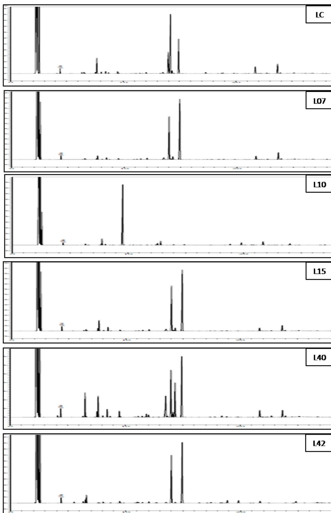
Figura 7- Cromatogramas fornecidos por análise em GC-FID do óleo essencial da Lippia alba comum (LC) e dos 6 acessos da coleção de Lippia spp da Embrapa
