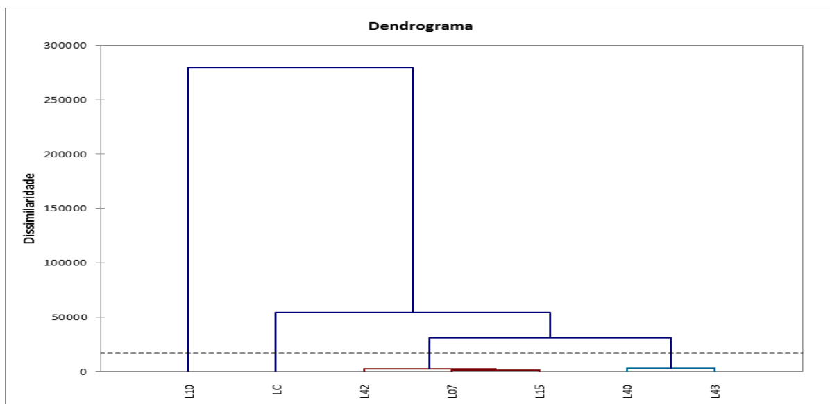
Figura 9 – Análise de agrupamento Hierárquico (clusters dos compostos voláteis (concentração em mg/mL) detectados no óleo essencial de genótipos de Lippia alba (Mill.) N. E. Brown do Banco de Germoplasma da Embrapa (DF), cultivadas no Horto de Plantas Medicinais da Embrapa (CE).
