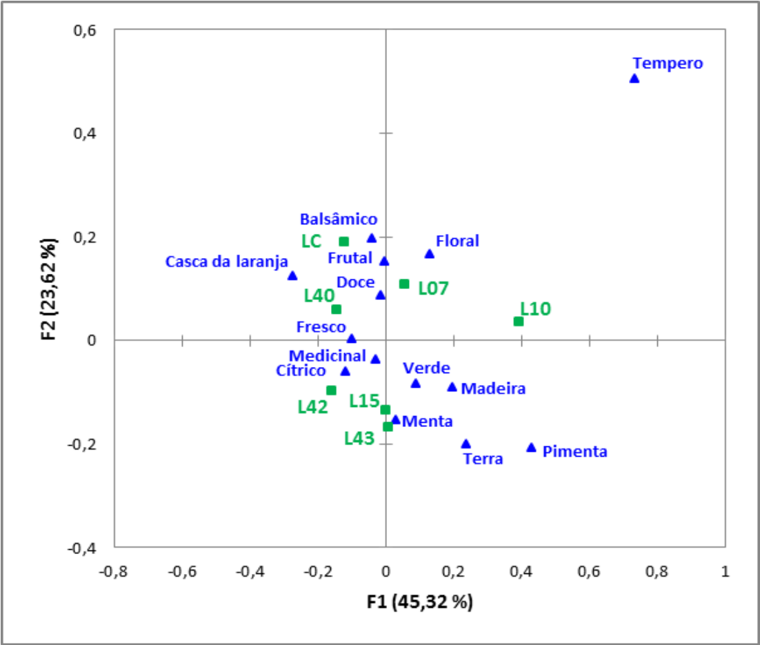
Figura 11. Gráfico simétrico gerado pela Análise de Correspondência dos dados do teste CATA para aroma dos óleos essenciais de Lippia alba .
