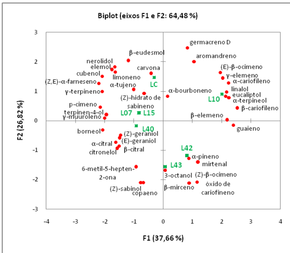
Figura 10 – Análise de Componentes Principais dos compostos voláteis detectados no óleo essencial de genótipos de Lippia alba (Mill.) N. E. Brown do Banco de Germoplasma da Embrapa (DF), cultivadas no Horto de Plantas Medicinais da Embrapa (CE).
