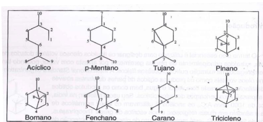
Figura 1. Estruturas básicas dos compostos monoterpênicos.
