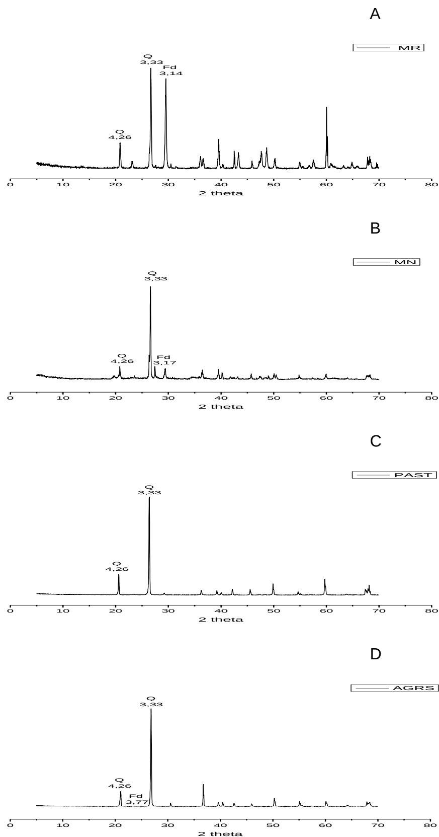
Figura 3.3 – Difractogramas de raios X da fração areia grossa dos sedimentos dos sistemas: A= mata raleada (MR), B= mata nativa (MN), C= pastagem (PAST) e D= agricultura de subsistência (AGRS). Minerais: Q= quartzo, Fd= feldspato.
