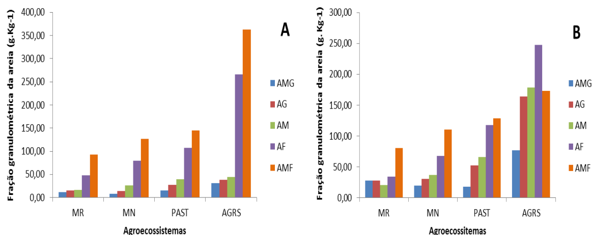
Figura 4.4 – Granulometria da fração areia de solos (A) e sedimentos de arraste (B) de agroecossistemas do semiárido de Iguatu. (AMG= Areia Muito Grossa; AG= Areia Grossa; AM= Areia Média; AF= Areia Fina e AMF= Areia Muito Fina).
