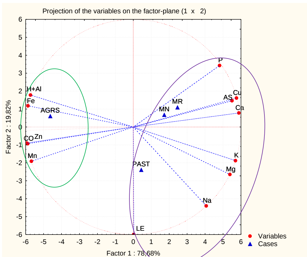
Figura 1.2 - Análise de componentes principal de atributos químicos e de perdas de sedimentos durante o período chuvoso de 2011 em agroecossistemas da região semiárida, Iguatu. (LE= lâmina de escoamento superficial; AS= produção de sedimentos de arraste; CO= carbono orgânico).
