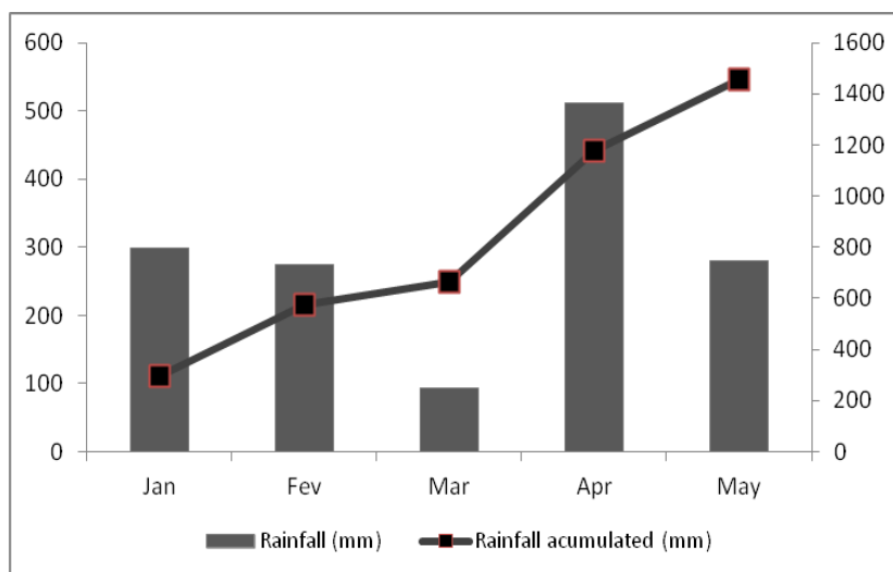
Figura 2.2 – Precipitação mensal em agroecossistemas de Iguatu e valores acumulados de janeiro a maio, 2011.
