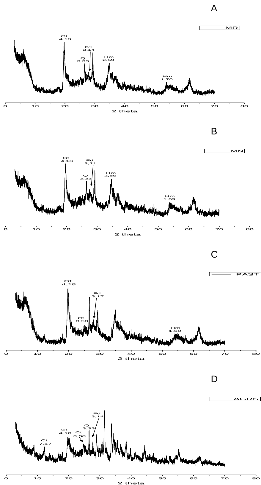
Figura 3.5 – Difrátogramas de raios X da fração argila natural dos sedimentos dos sistemas: A= mata raleada (MR), B= mata nativa (MN), C= pastagem (PAST) e D= agricultura de subsistência (AGRS). Minerais: Qz= quartzo, Fd= feldspato, Gt= goethita, Hm= hematita, Ct= caulinita.
