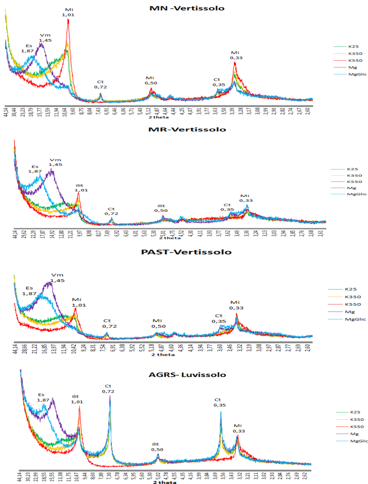
Figura 3.6 – Difrátogramas de raios X da fração argila desferrificada, saturada com K e aquecida a temperatura de 25 (K25), 350 (K350) e 550°C (K550), saturada com Mg (Mg) e Mg+glicerol (MgGlic) dos sedimentos dos sistemas de mata raleada (MR), mata nativa (MN), pastagem (PAST) e agricultura de subsistência (AGRS). Minerais: Es= esmectita, illit= illita, Mi= mica, Vm= vermiculita, Ct= caulinita.
