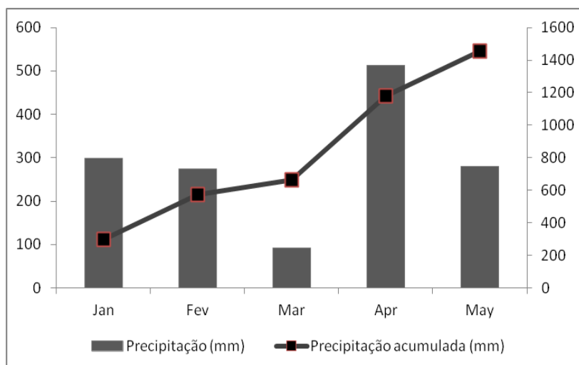
Figura 3.2 – Precipitação mensal e acumulada de janeiro a maio de 2011 nos agroecossistemas de Iguatu, estado do Ceará.
