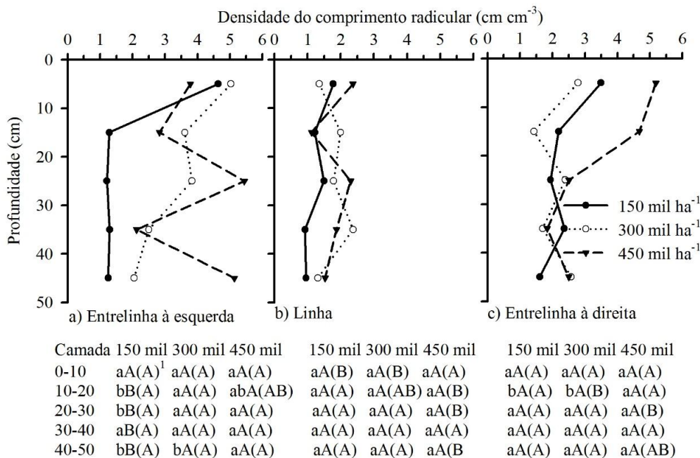
Figura 5. Densidade do comprimento radicular, cultivar BRS 359 RR, em diferentes camadas de solo, posições de amostragem e densidades de plantas. Londrina, PR, safra 2014/2015.
