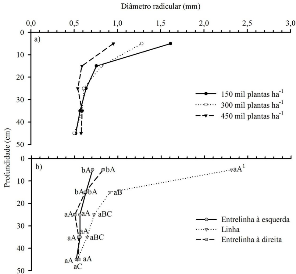
Figura 7. Diâmetro de raízes ponderado pelo comprimento (mm), cultivar BMX Potência RR, em diferentes camadas de solo em função da densidade de plantas (a) e posições de amostragem (b). Londrina, PR, safra 2014/2015.
