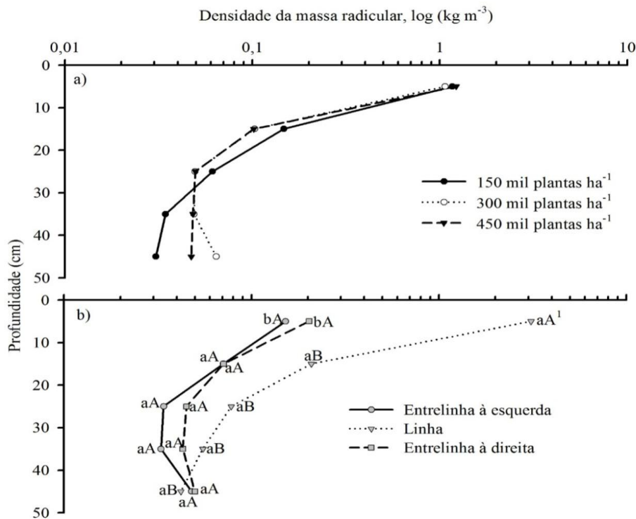
Figura 3. Densidade de massa radicular de soja (eixo x em escala log), cultivar BMX Potência RR, em diferentes camadas de solo em função da densidade de plantas (a) e posições de amostragem (b). Londrina, PR, safra 2014/2015.
