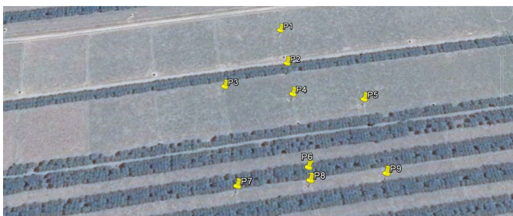
Figura 2. Posições espaciais de medida de microclima no bloco 2 do experimento de ILPF-Leite da Embrapa Agrossilvipastoril, Sinop, MT.
