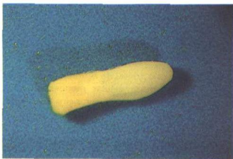
FIG. 1a. Embrião de caiaué. Comprimento 3 mm e aproximadamente x 16.
