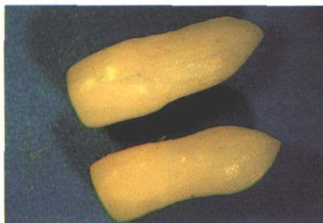
FIG. 1b. Embriões de híbrido. Comprimento 3 mm e aproximadamente x 16.
