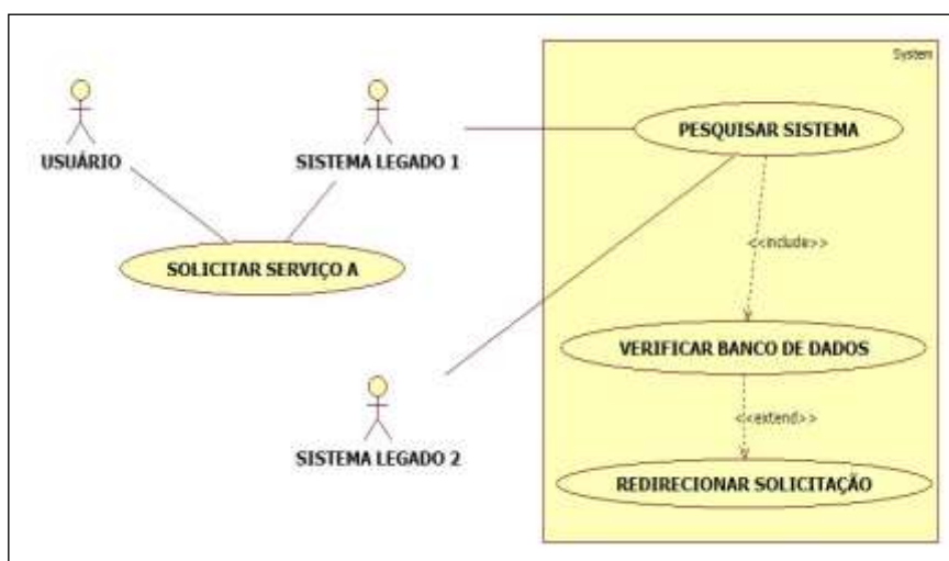
Figura 2 – Diagrama de caso de uso proposto
