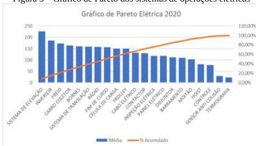
Figura 3 – Gráfico de Pareto dos sistemas de operações elétricas
