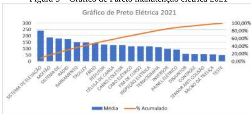
Figura 5 – Gráfico de Pareto manutenção elétrica 2021
