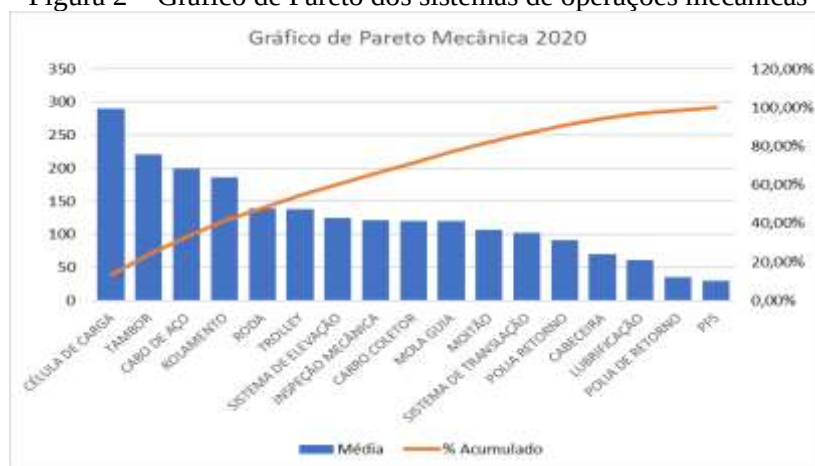
Figura 2 – Gráfico de Pareto dos sistemas de operações mecânicas
