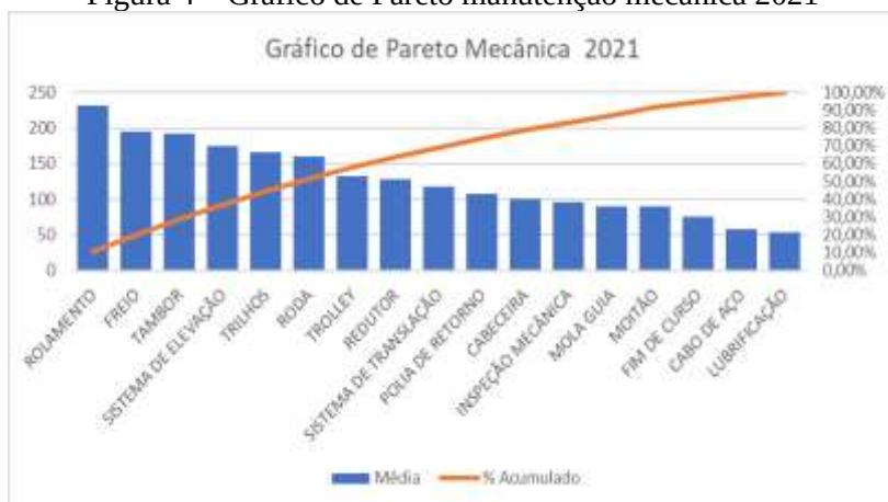
Figura 4 – Gráfico de Pareto manutenção mecânica 2021
