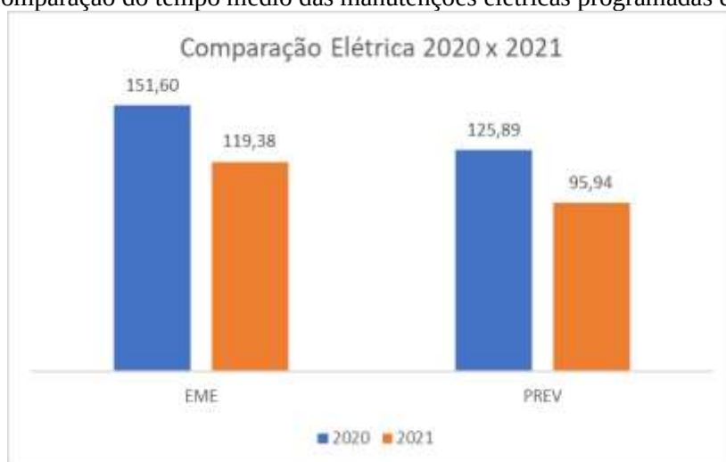
Figura 7 – Comparação do tempo médio das manutenções elétricas programadas e emergenciais
